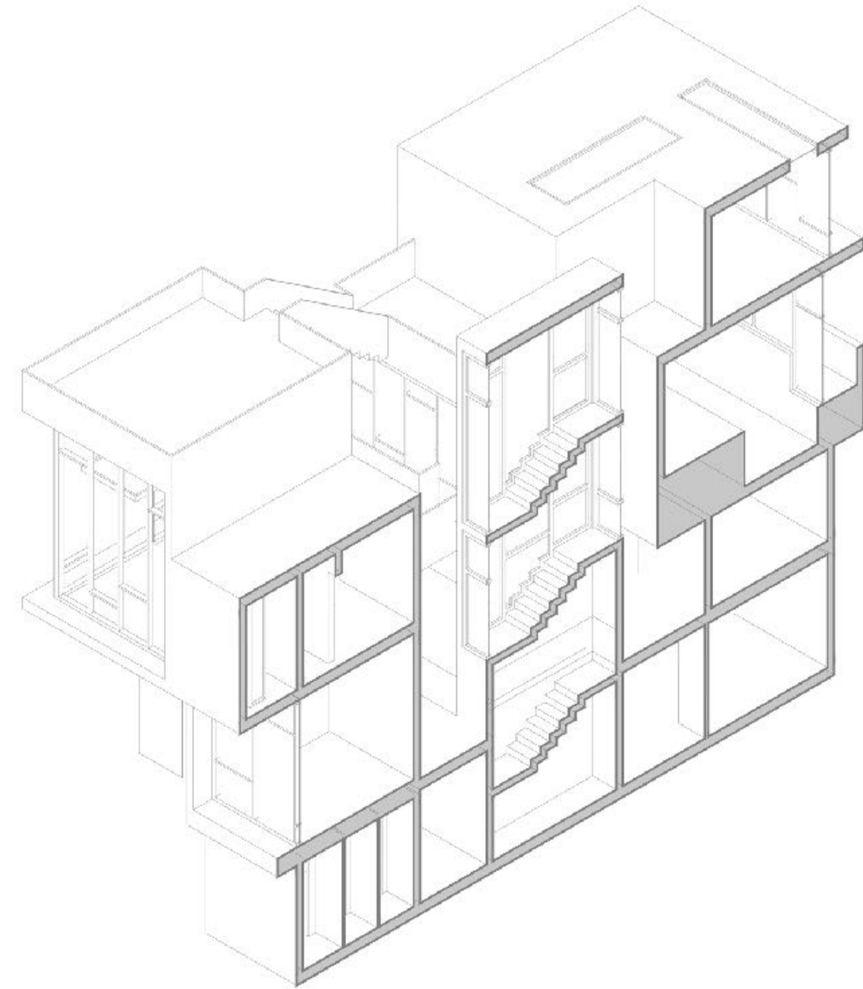
3 ISO SEC C Scale: 1:100
