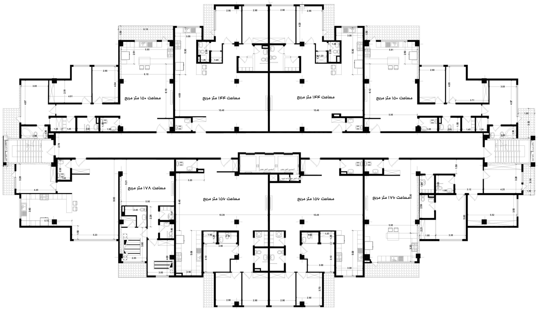
پلان اندازه گذاری طبقات ۸ واحدی
