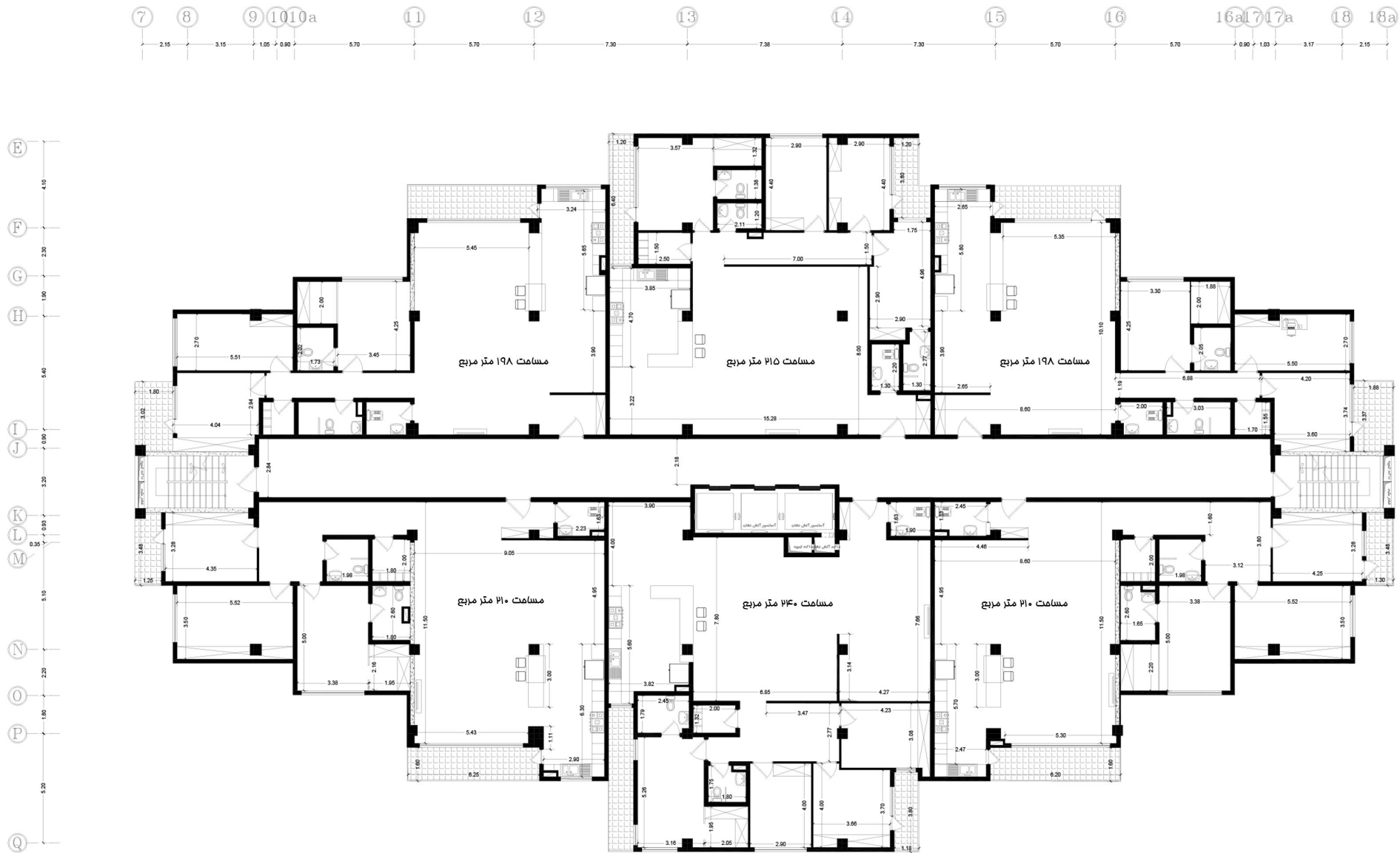
پلان اندازه گذاری گذاری طبقات ۶ واحدی
