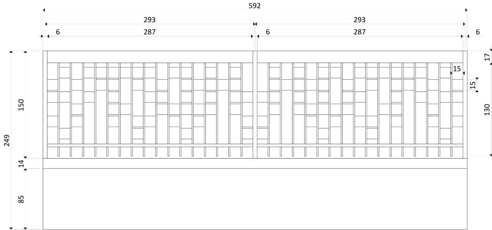
● نمای شمالی
