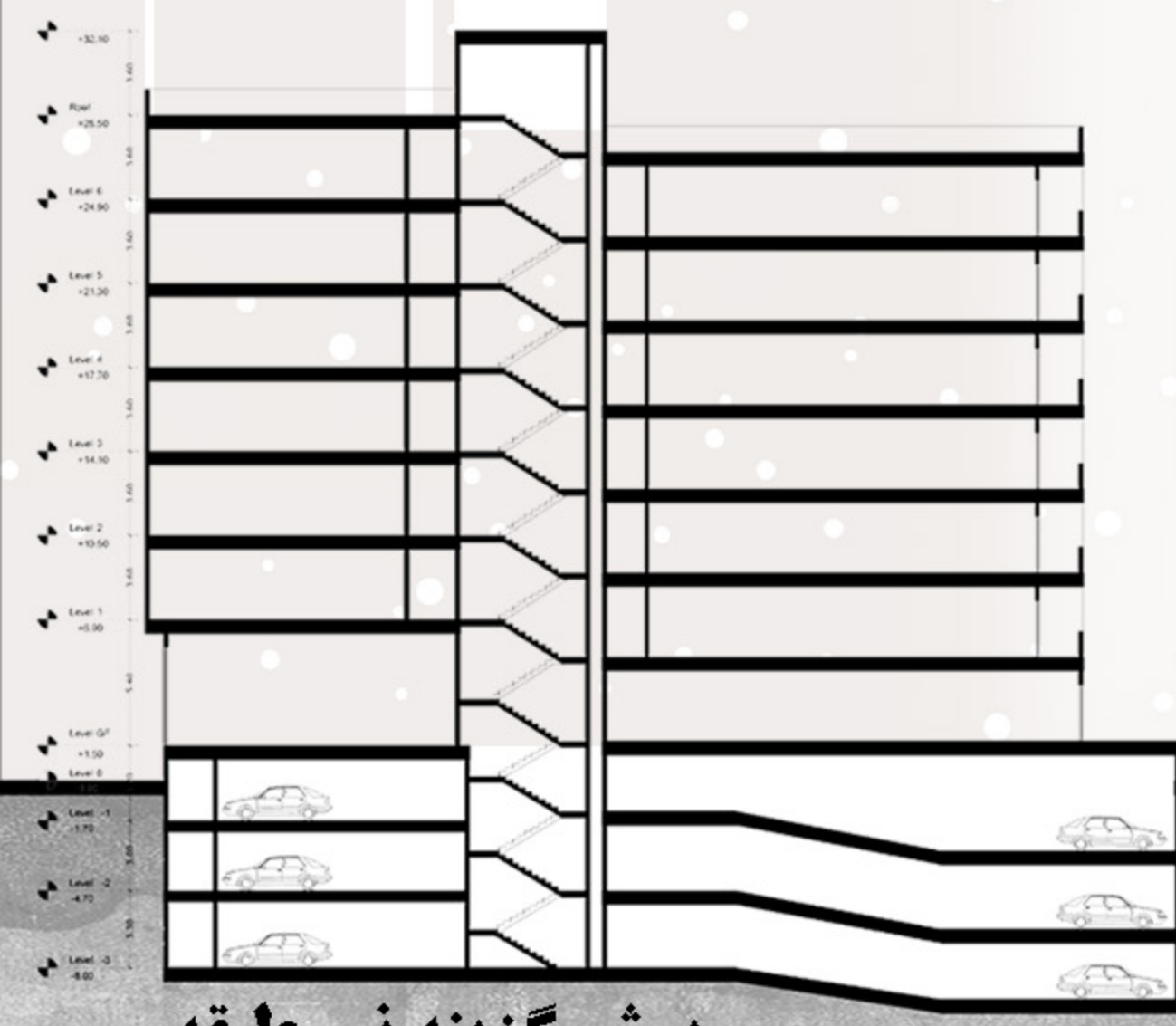
برش گزینه نیم طبقه
