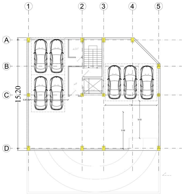
پلان زیرزمین ۱-
