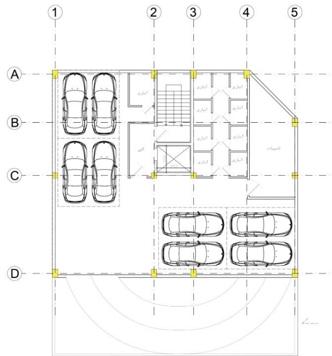
پلان زیرزمین ۲-
