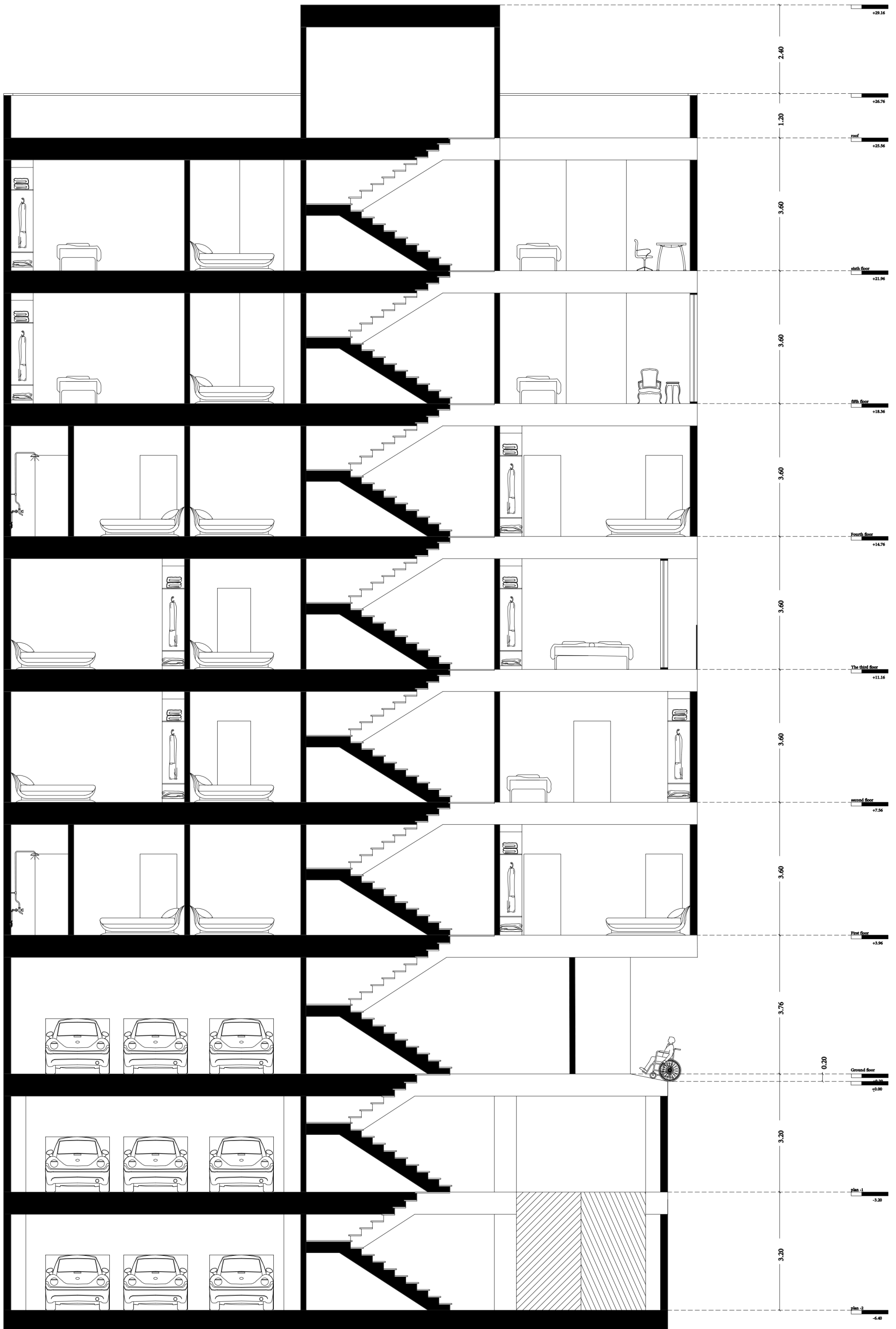
section A-A
