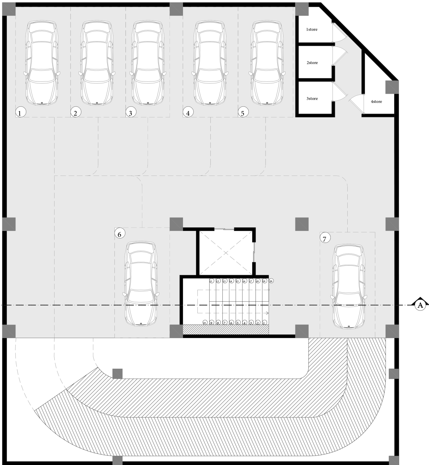
plan -2
