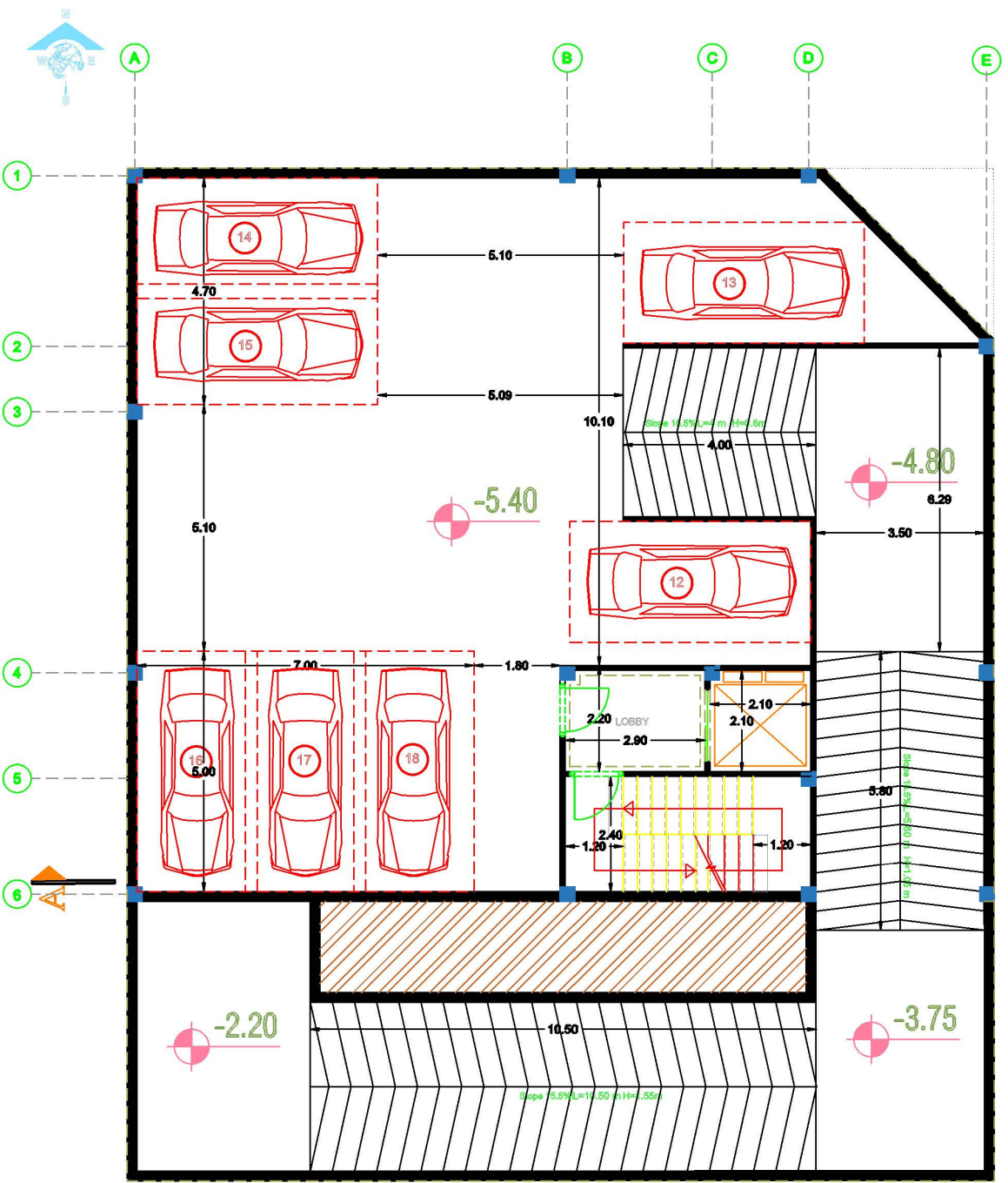
-2 Floor Dimension Plan Scale : 1\100
