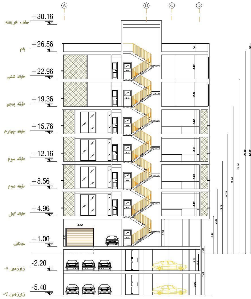
A-A مقطع Sc : 1/100
