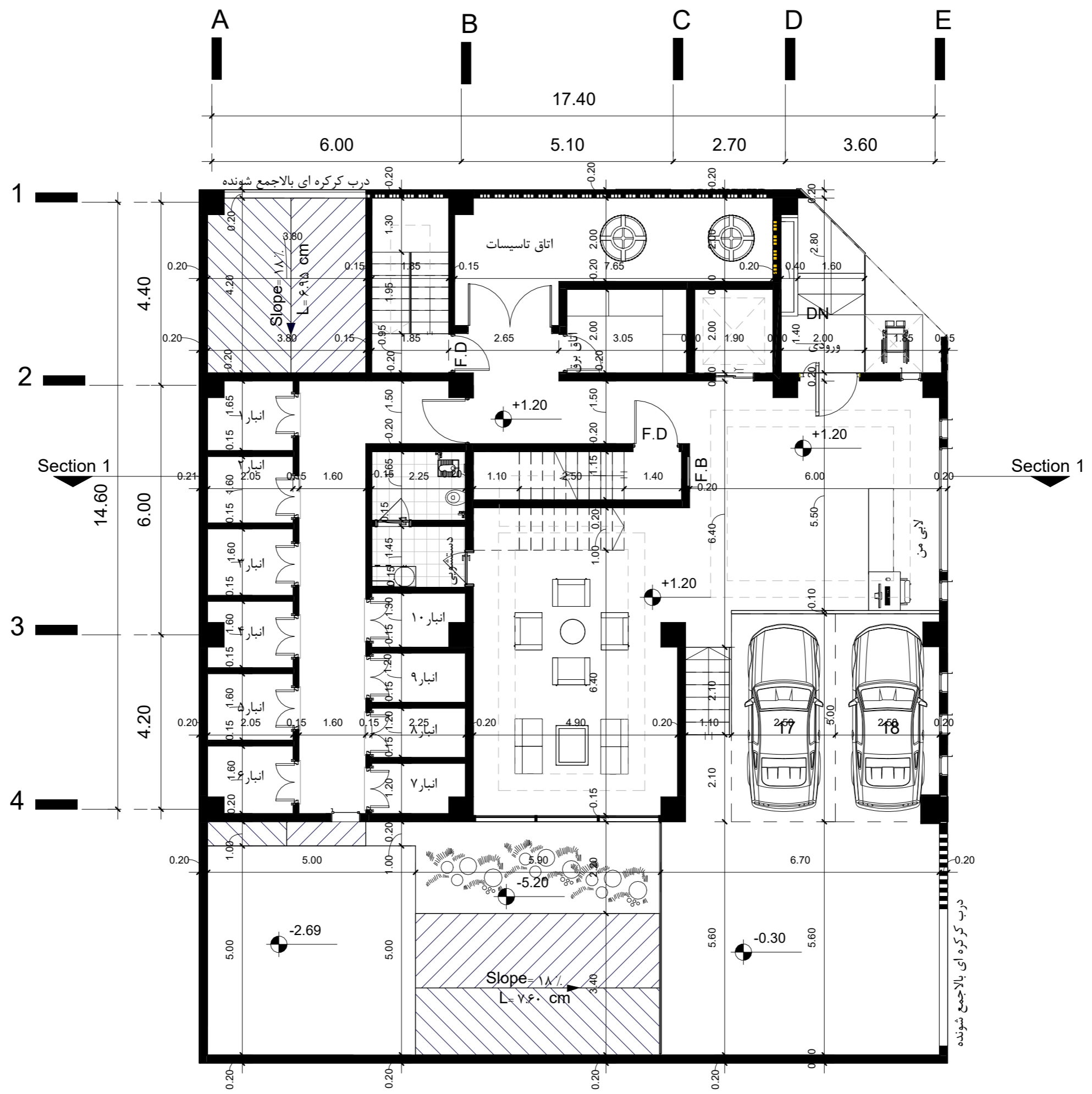
اندازه گذاری همگف SC: 1 : 100
