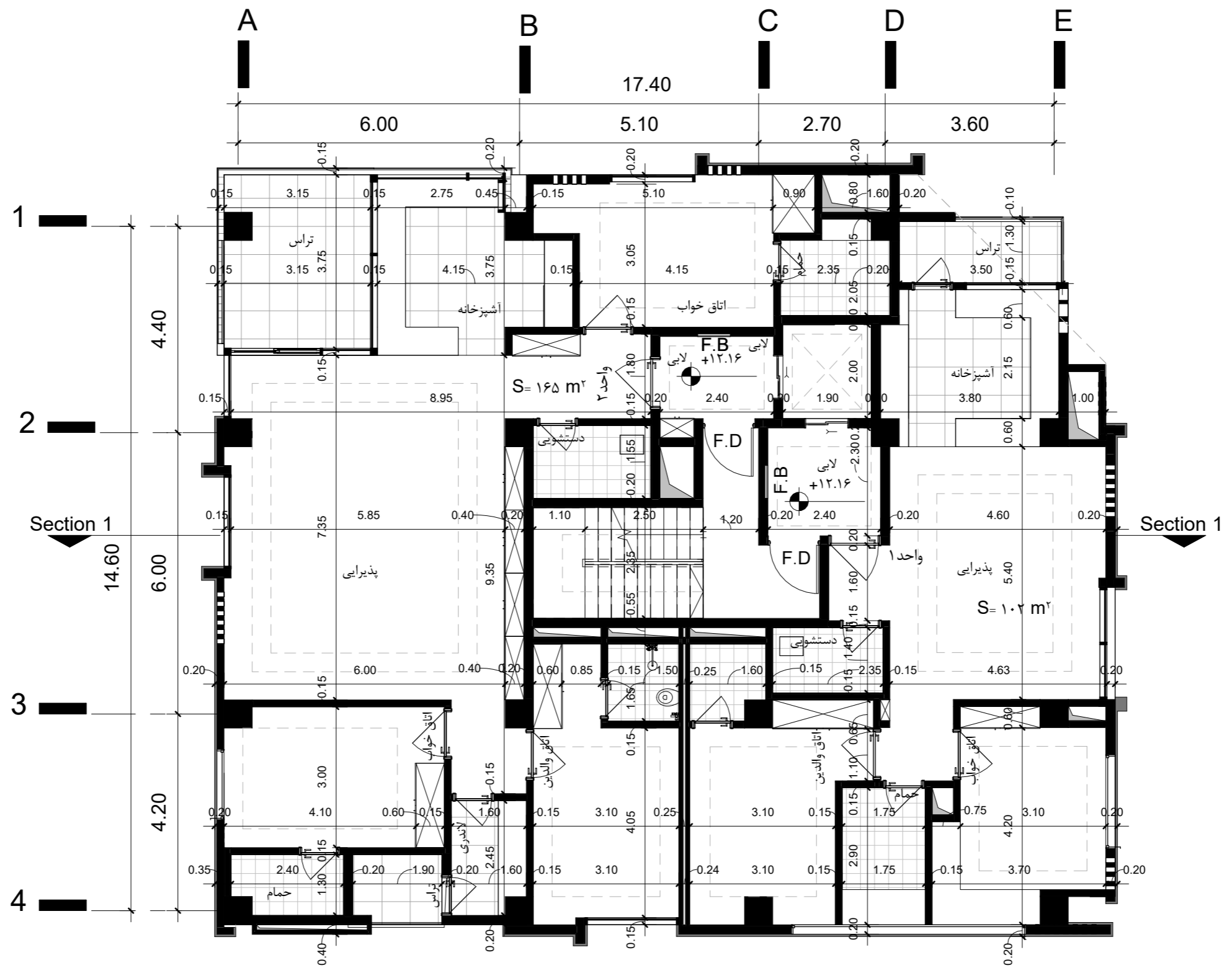
پلان اندازه گذاری طبقه سوم SC.1 : 100
