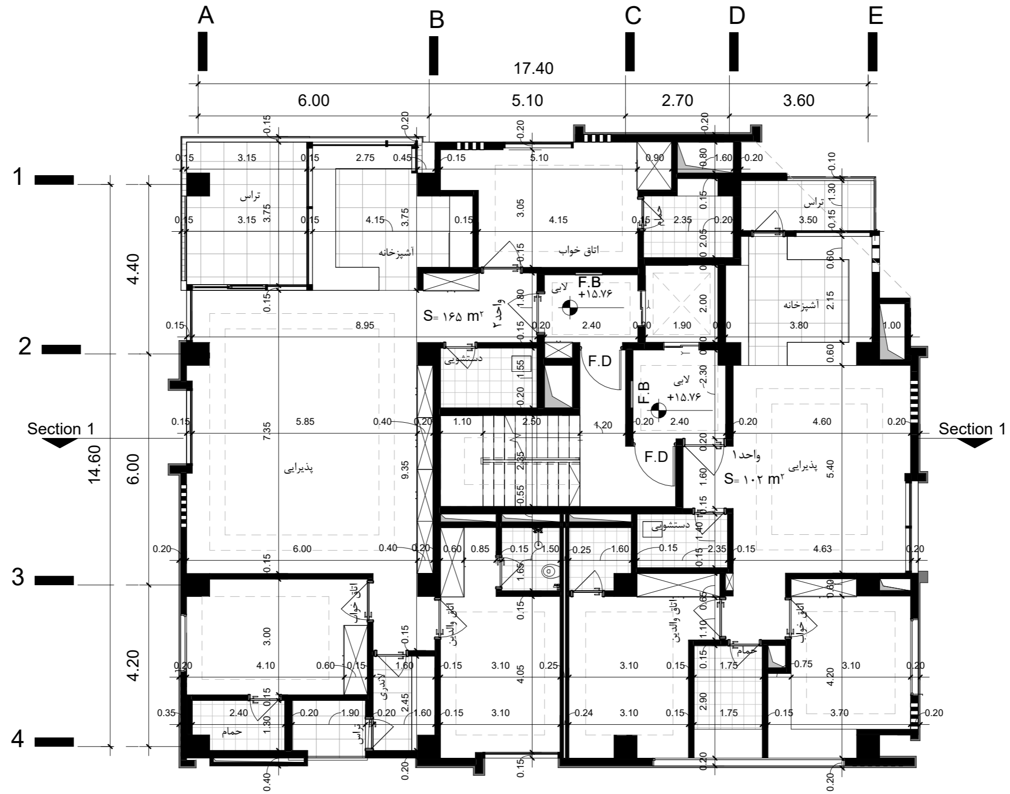
پلان اندازه گذاری طبقه چهارم SC:۱ : ۱۰۰
