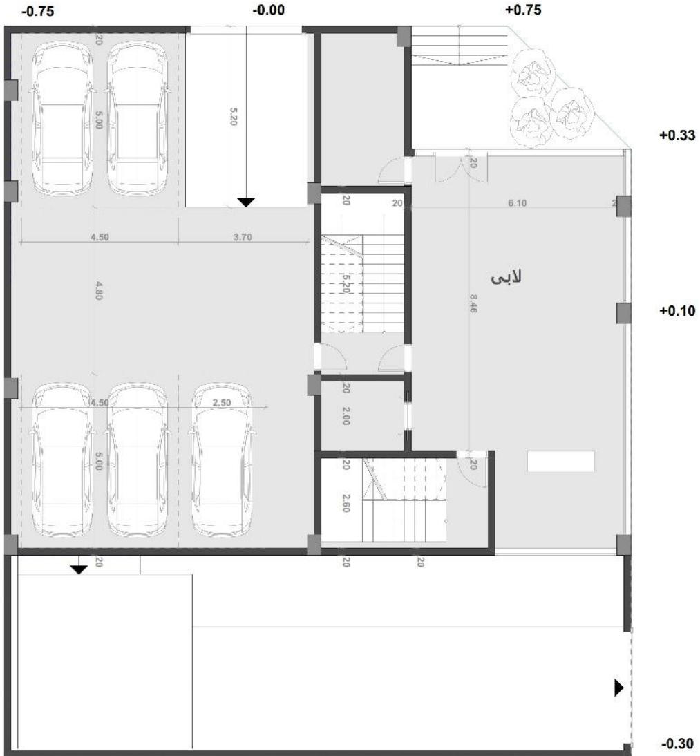
طبقه همکف
