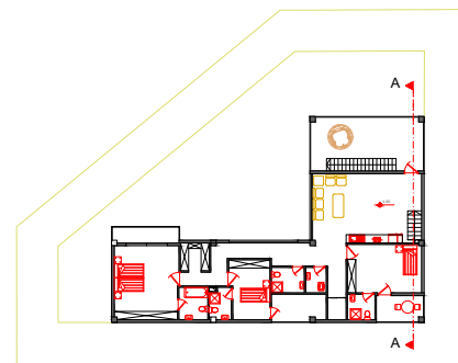
پلان طبقه دوم مساحت 209m
