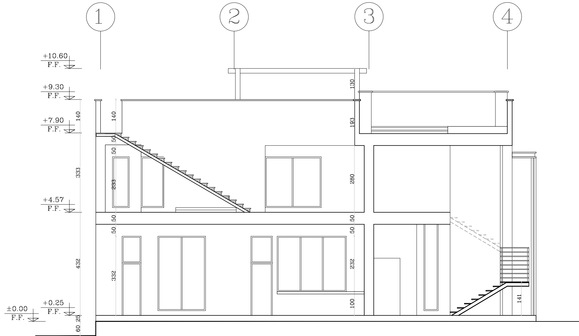
SECTION A-A
