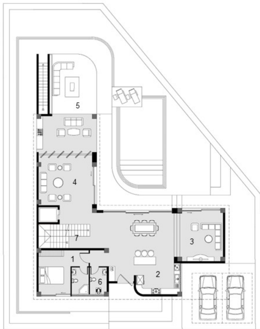
پلان همکف مساحت: ۲۰۶ مترمربع
