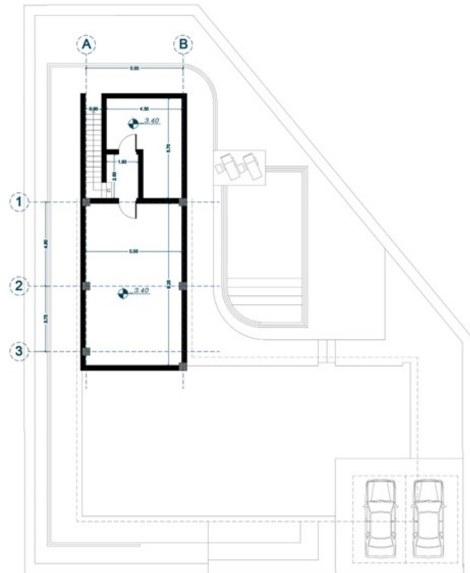
پلان اندازه گذاری زیرزمین
