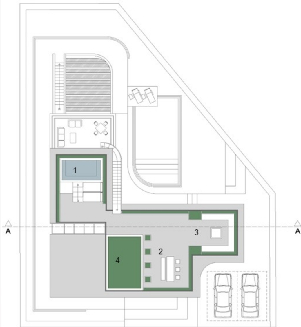
پلان روف گاردن مساحت: ۱۲۸.۳ مترمربع
