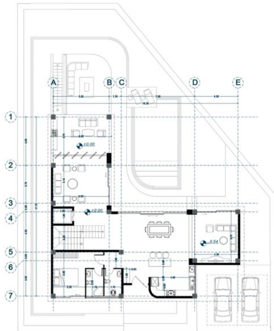
پلان اندازه گذاری همکف
