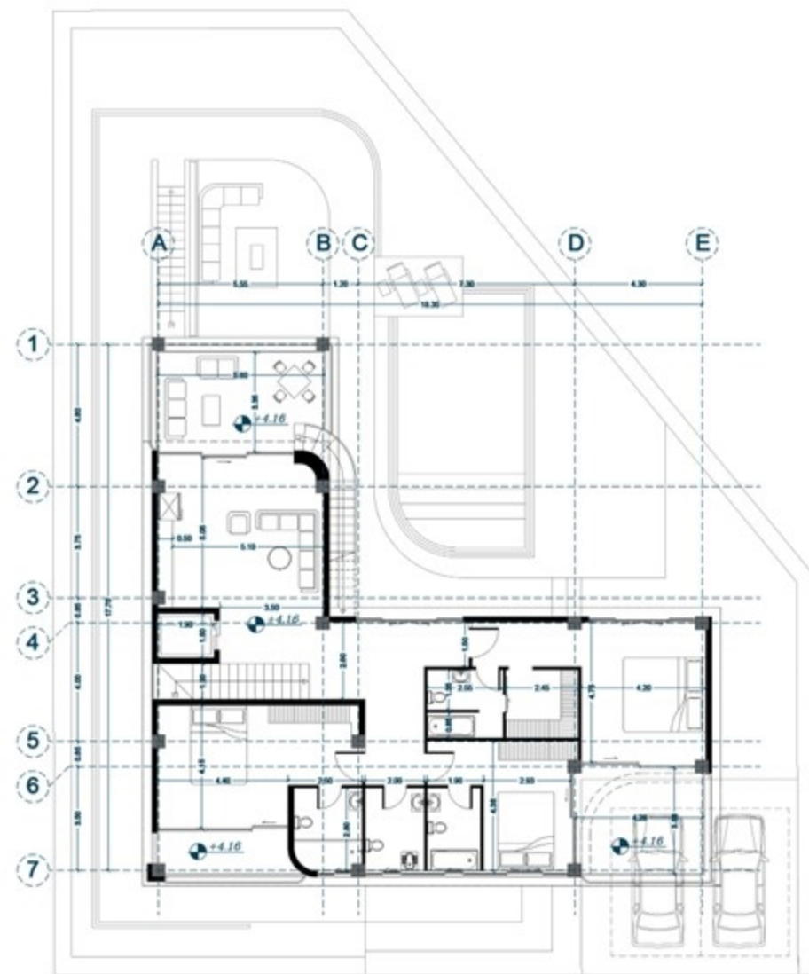
پلان اندازه گذاری طبقه اول
