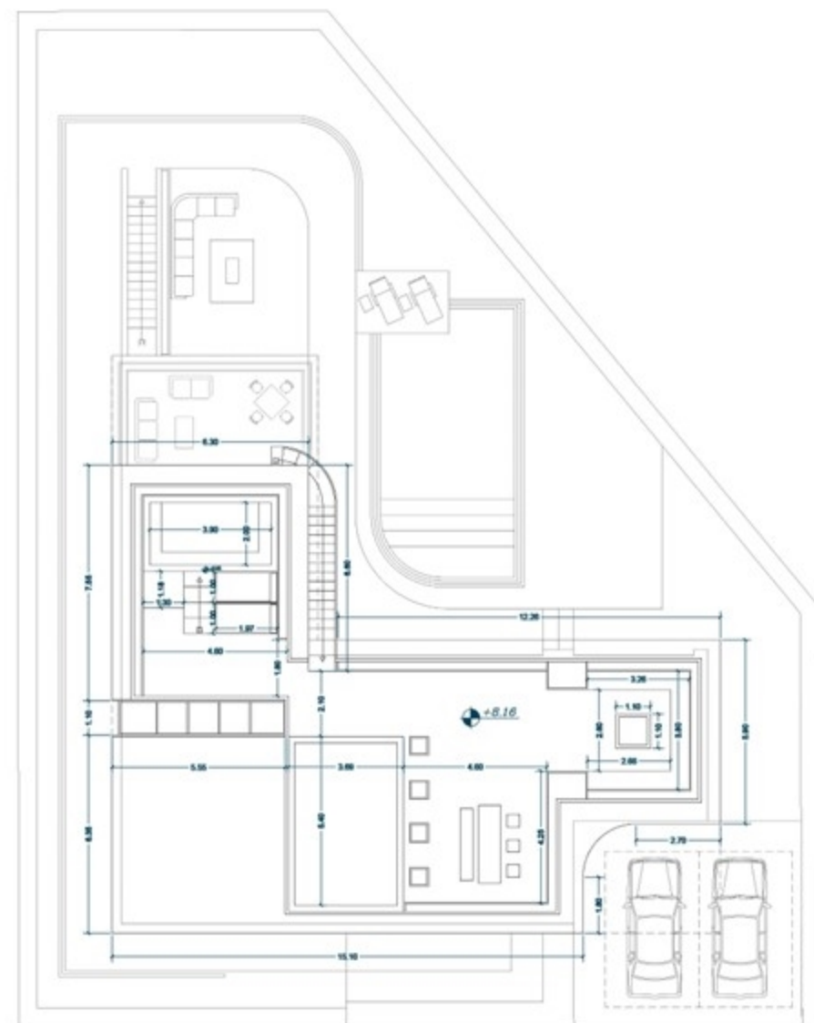
پلان اندازه گذاری روف گاردن
