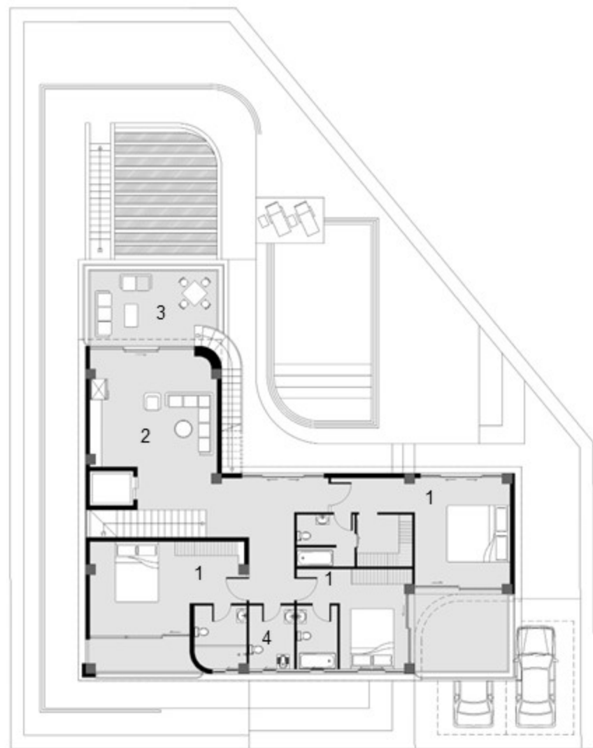
پلان اول مساحت: ۱۸۴.۳ مترمربع
