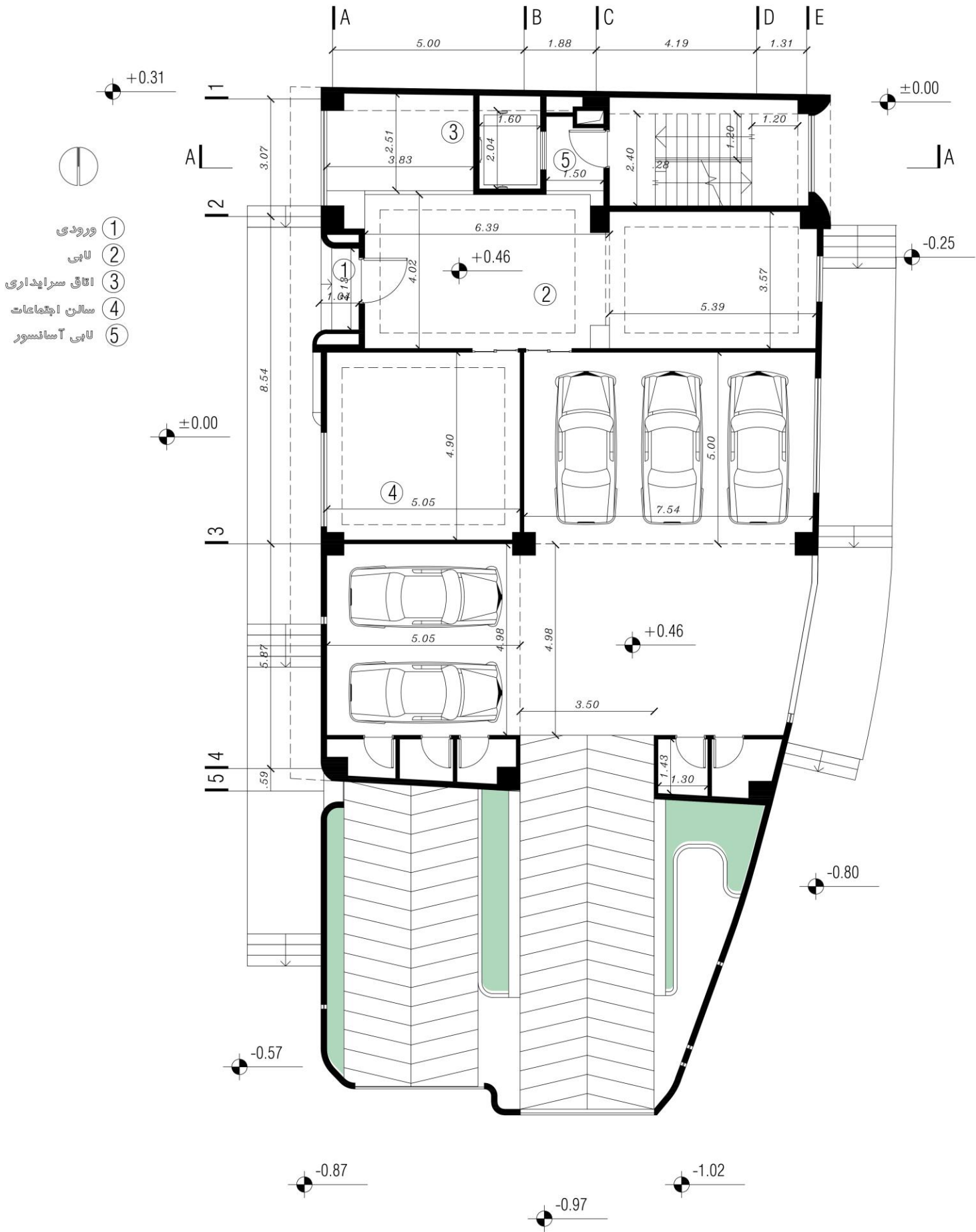
پلان اندازه گذاری طبقه همکف
