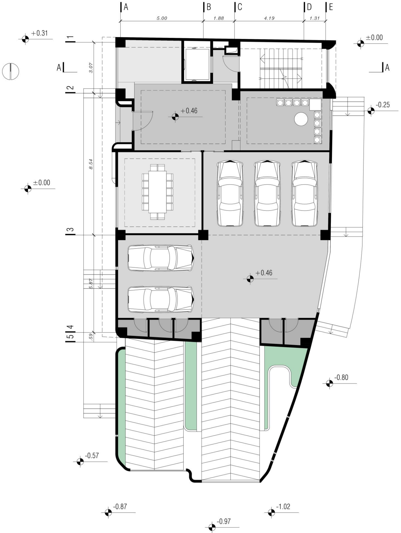
پلان میلمان طبقه همکف
