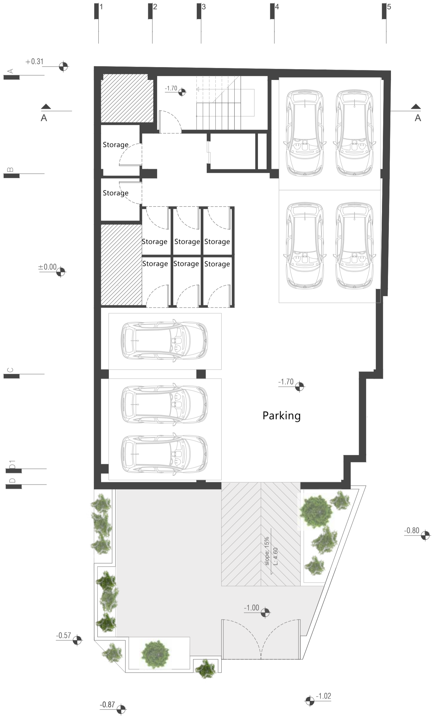
Basement Plan SC : 1/100
