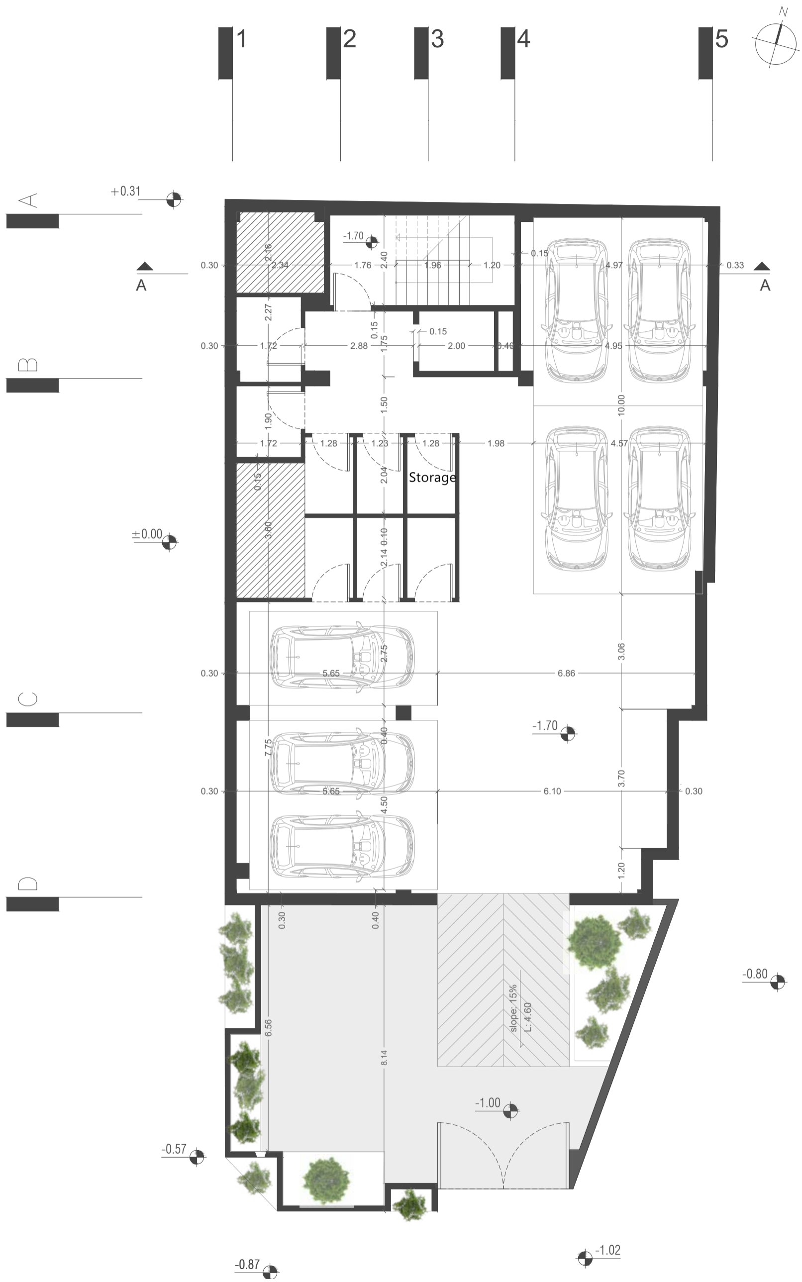
Basement Plan SC : 1/100
