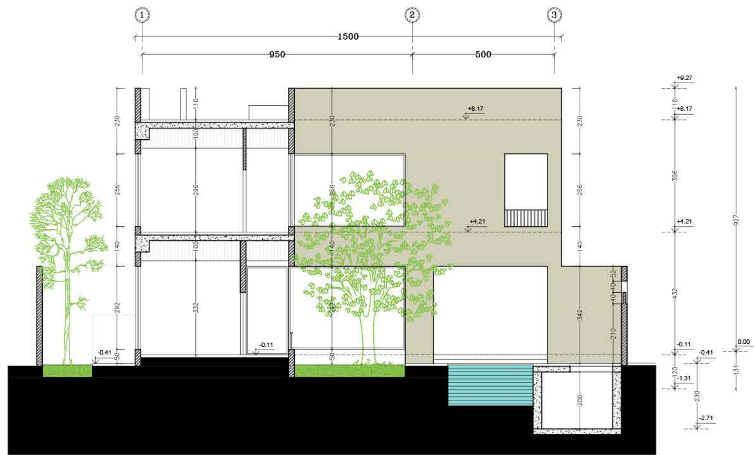
نما برش H-H
