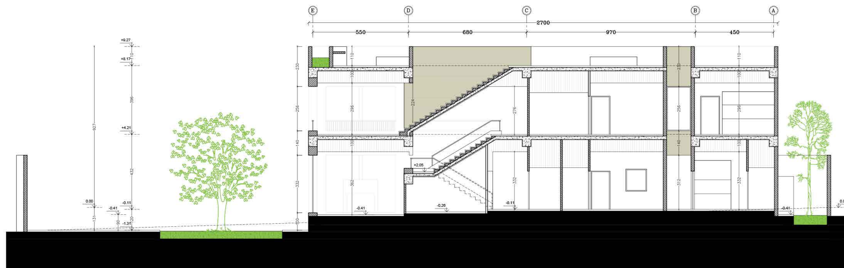
نما برش D-D
