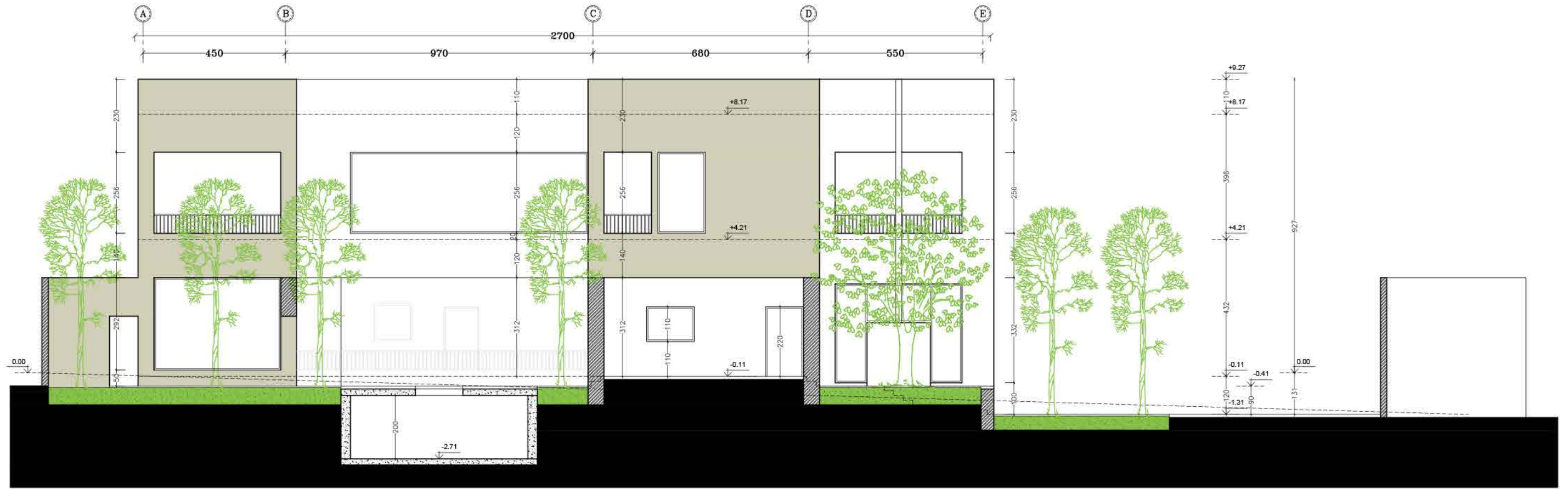
نما برش A-A
