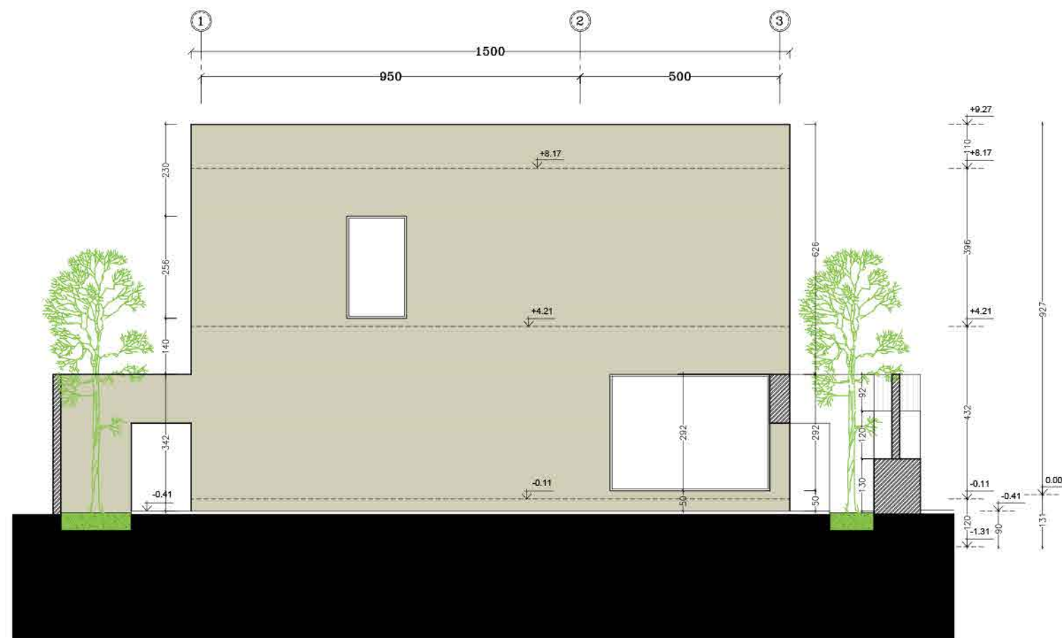
نما برش K-K
