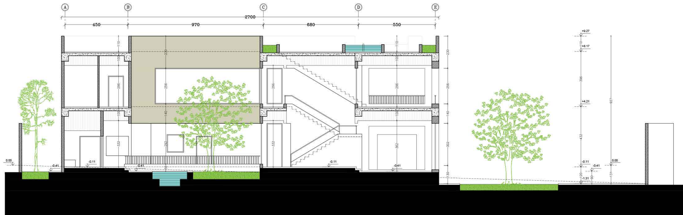
نما برش C-C
