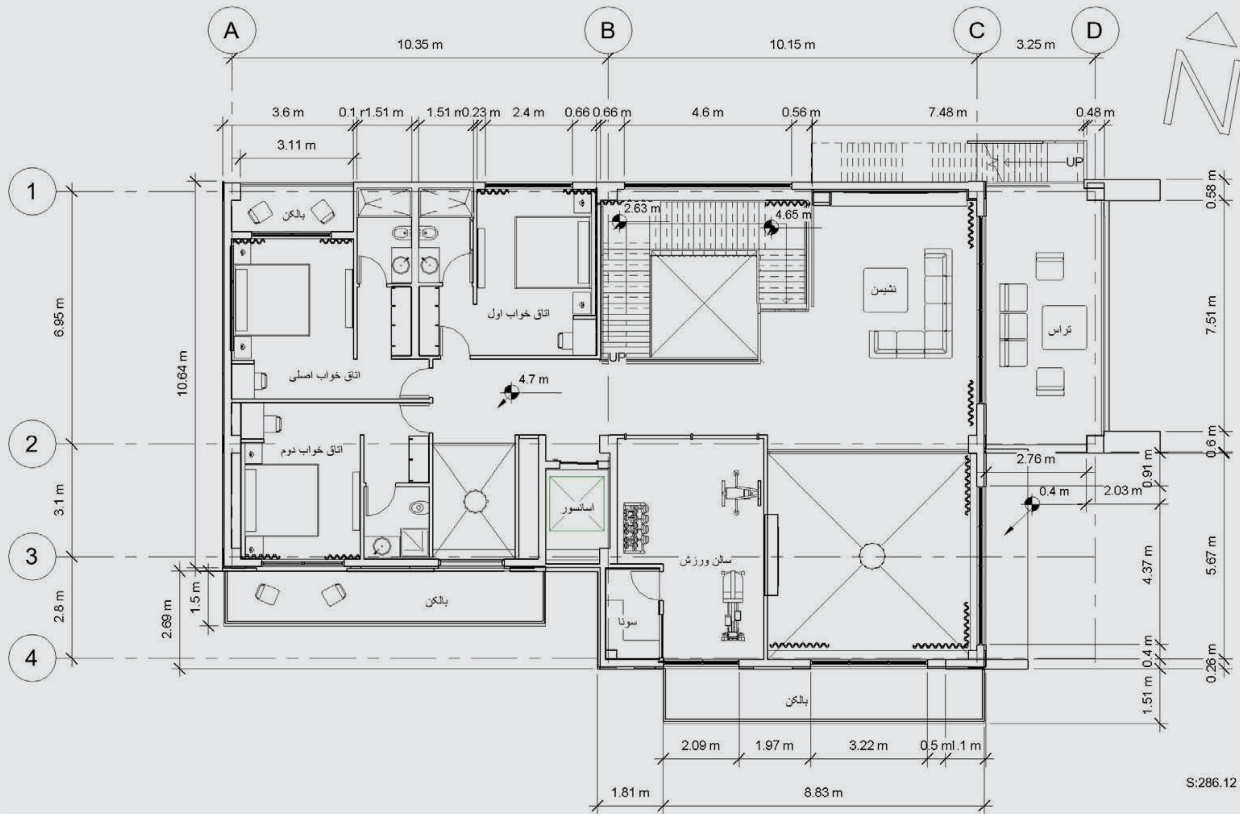
پلان طبقه اول اندازه گذاری
