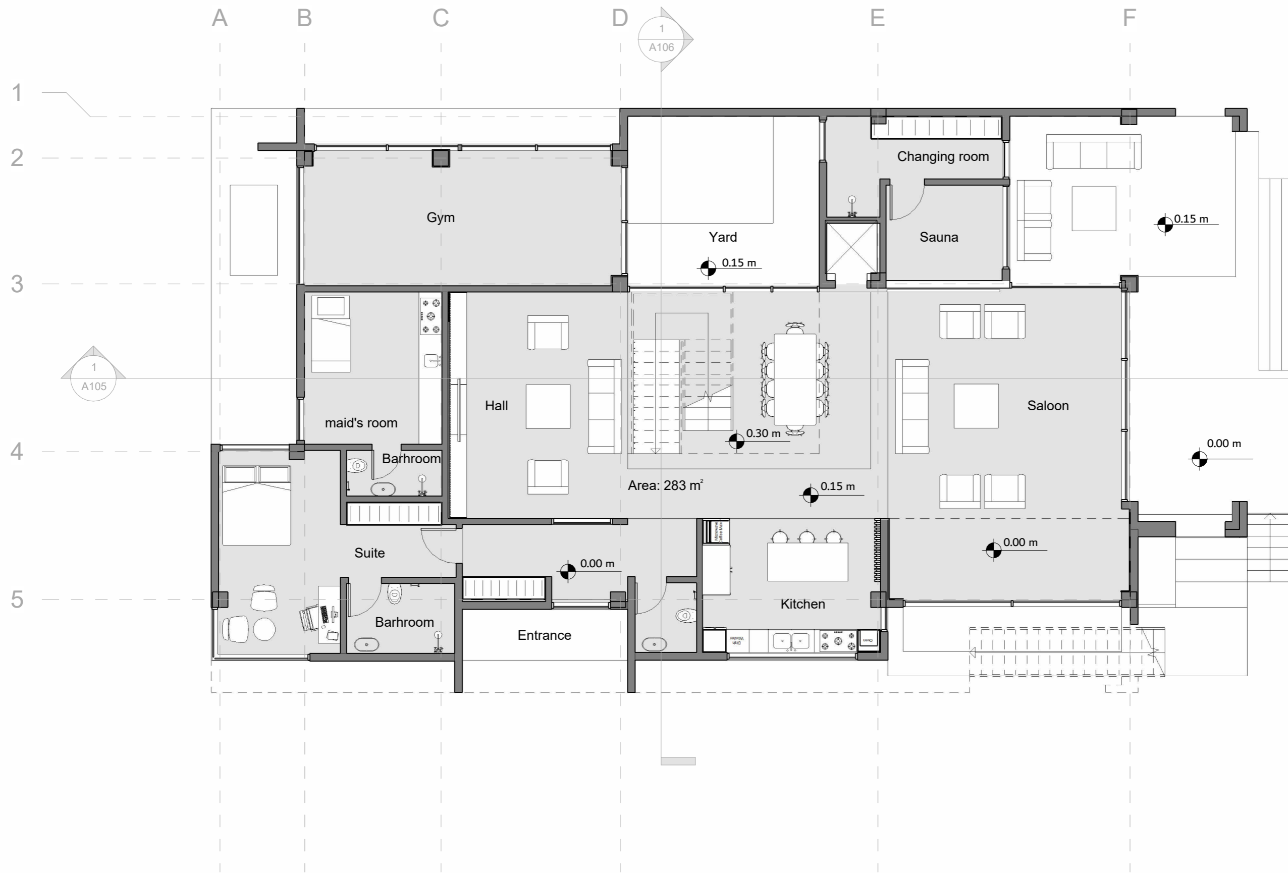
پلان طبقه همکف
