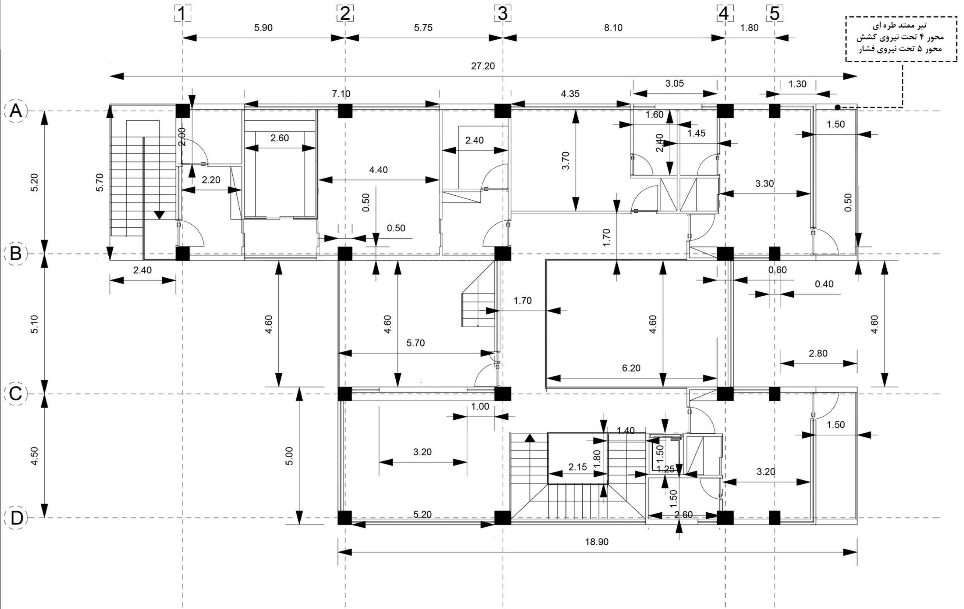
پلان ستون گذاری و اندازه گذاری طبقه اول، ارتفاع کف: ۸۰:۴ متر
