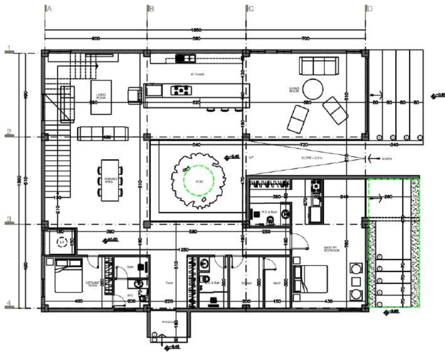
پلان معماری طبقه همکف
