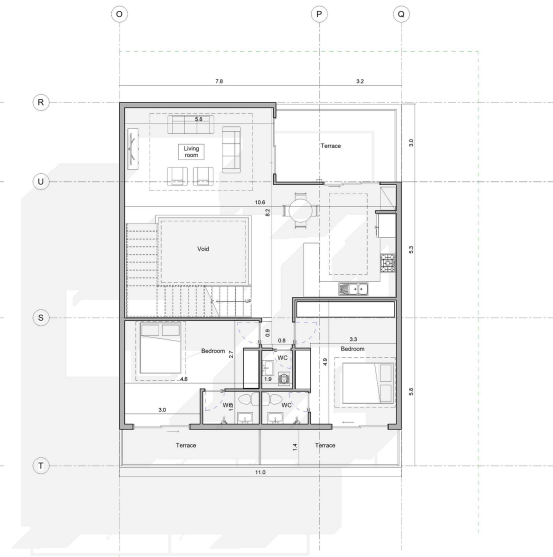
پلان اندازه گذاری طبقه اول
