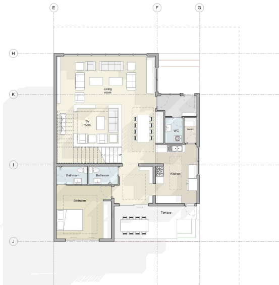
پلان مبلمان طبقه همکف
