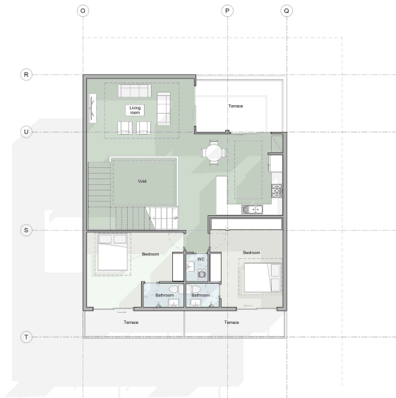
پلان مبلمان طبقه اول
