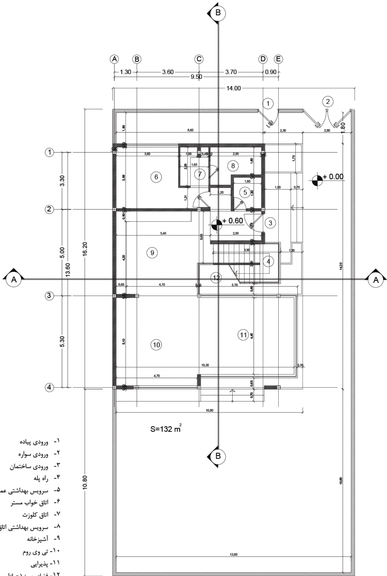
پلان اندازه گذاری طبقه همکف
