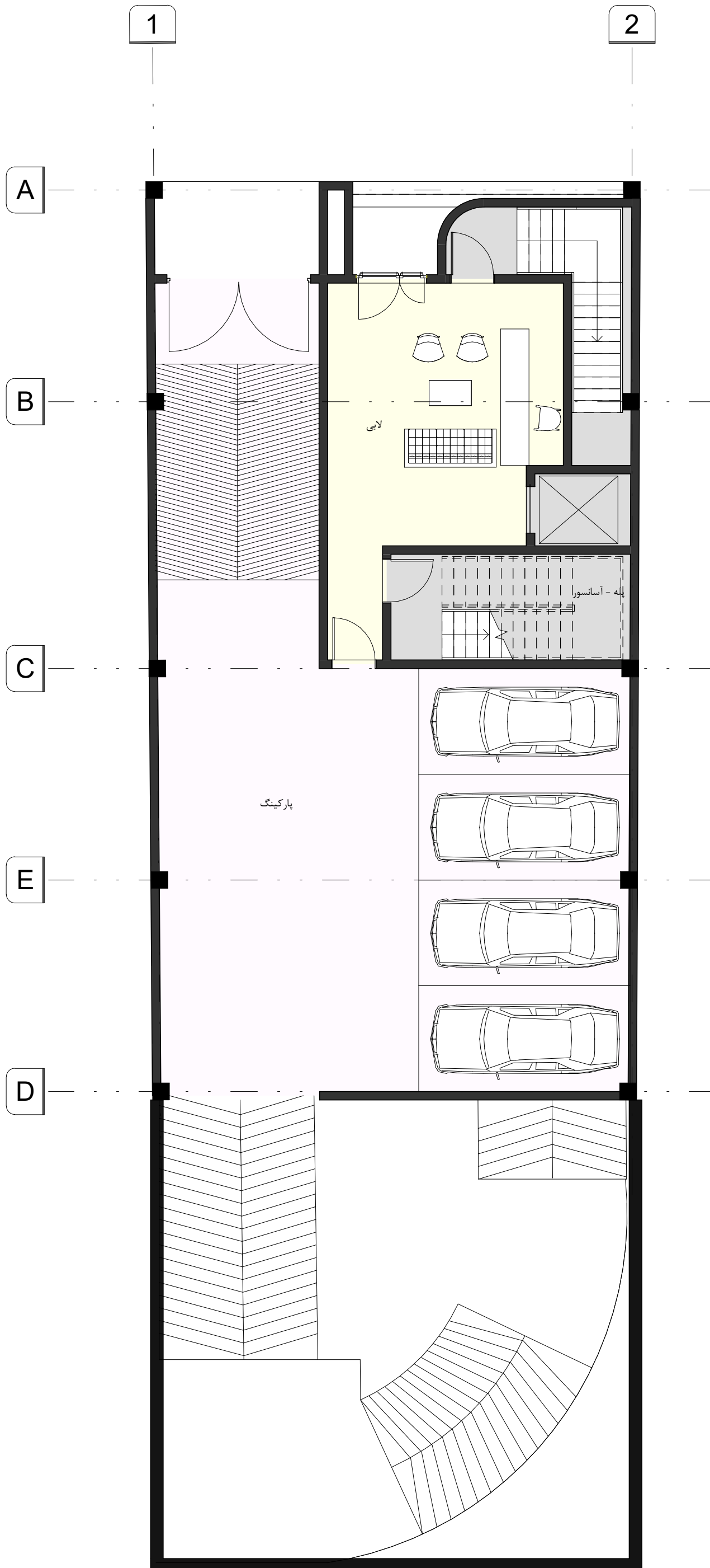
پلان میلمان همکف
