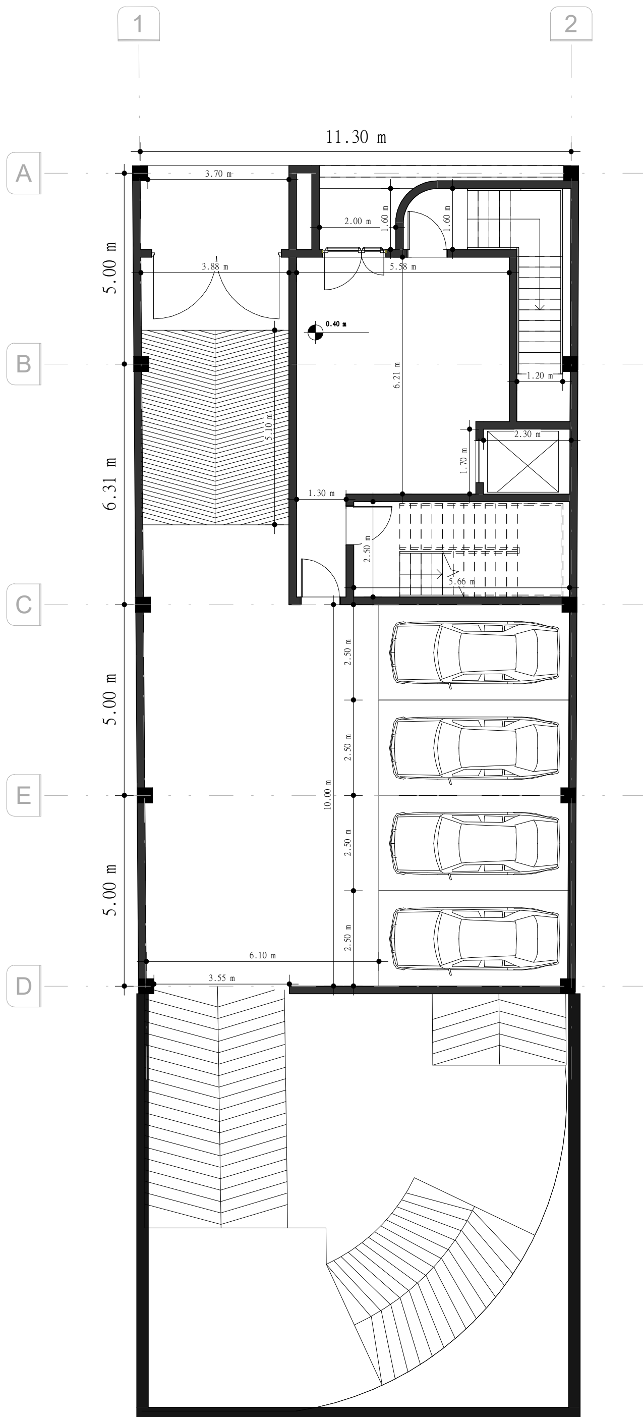
پلان اندازه گذاری همکف
