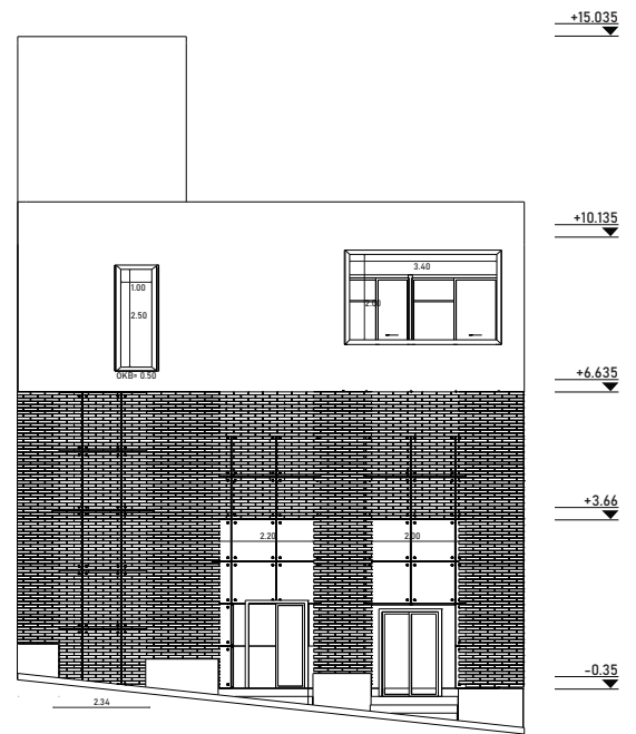
نما غربی مقیاس: ۱/۲۰۰
