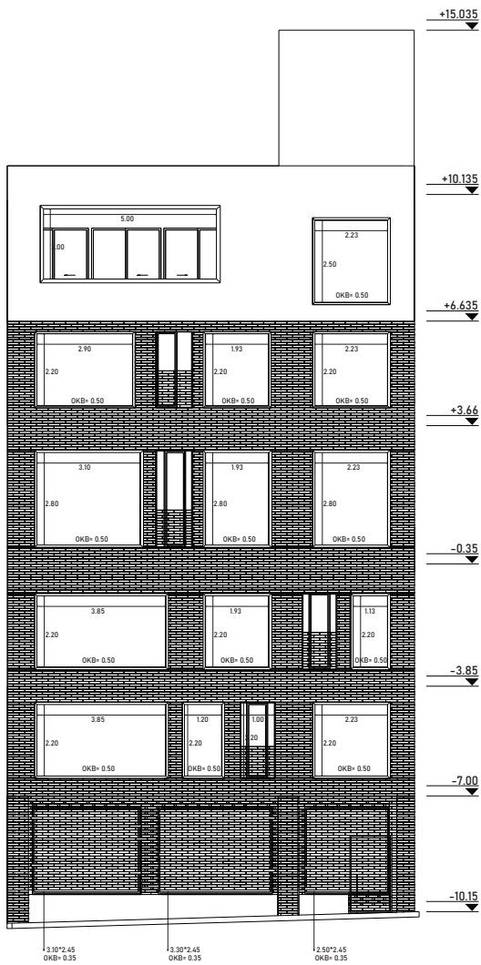
نما شرقی مقیاس: ۱/۲۰۰
