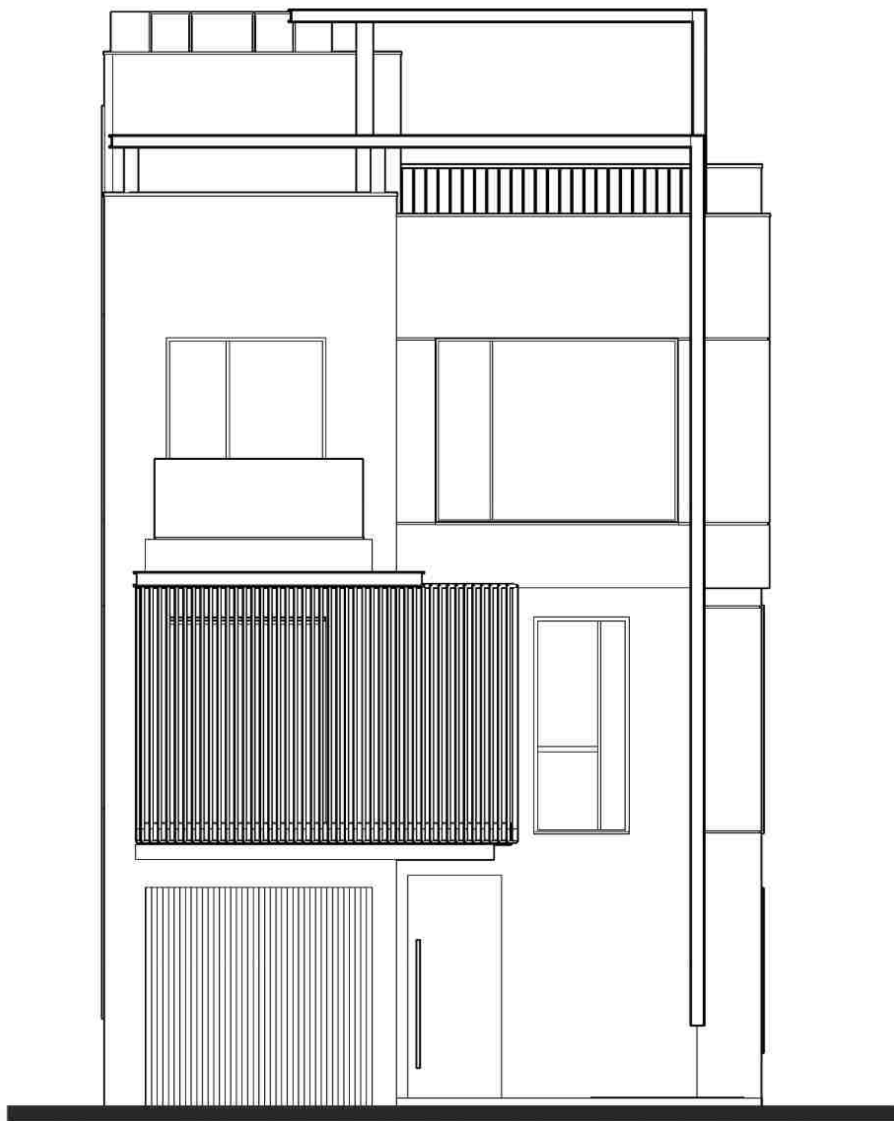
نمای شمالی
