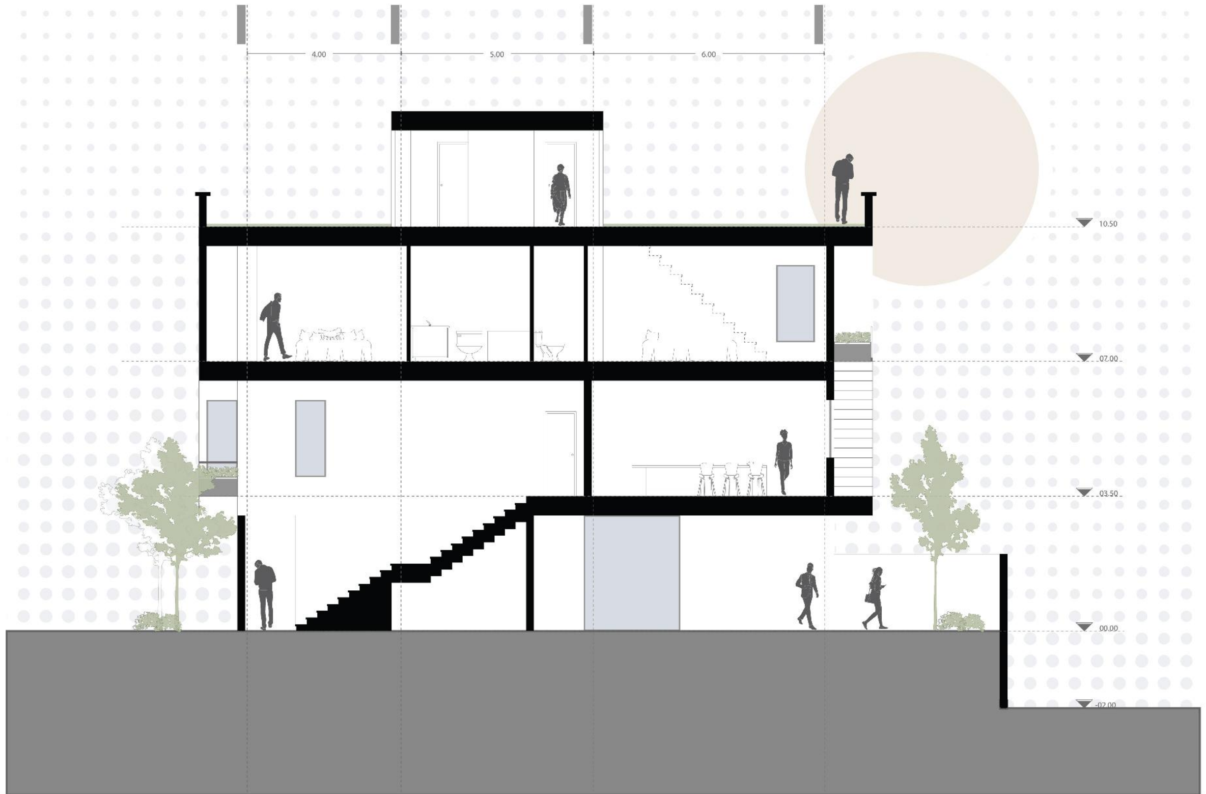
Section A-A
