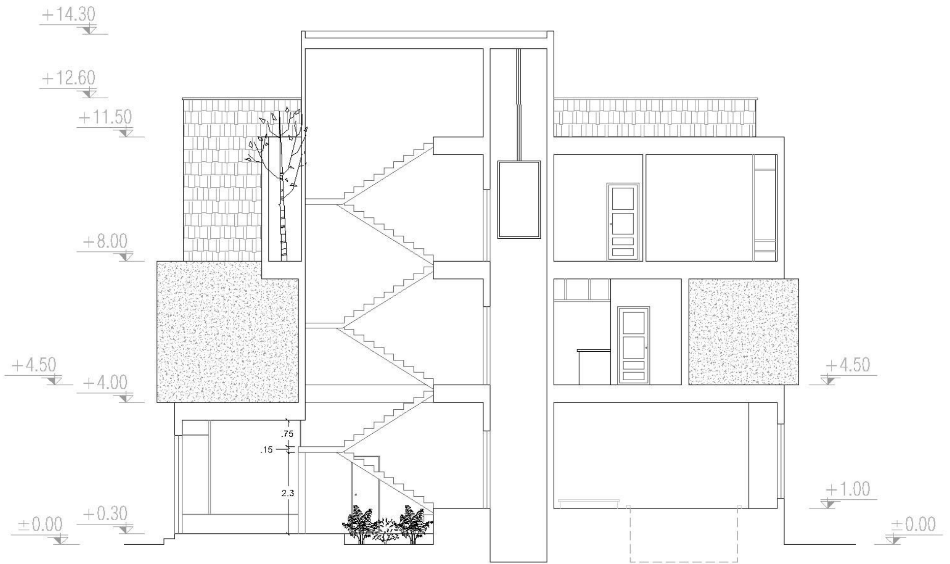
B-B برش مقیاس: 1:100
