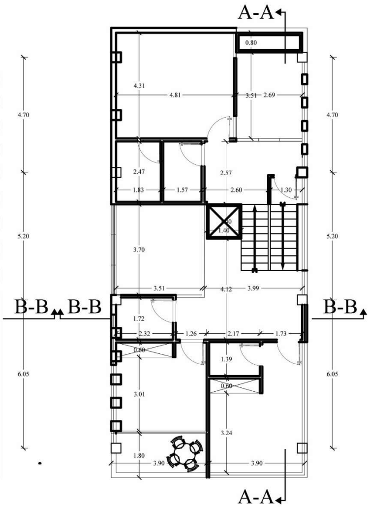
پلان طبقه دوم
