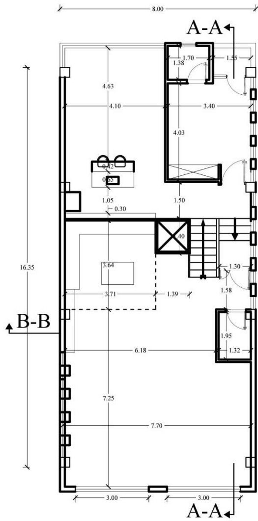
پلان طبقه اول
