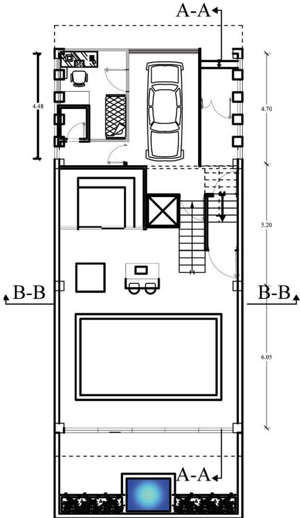
پلان آترناتیو همکف
