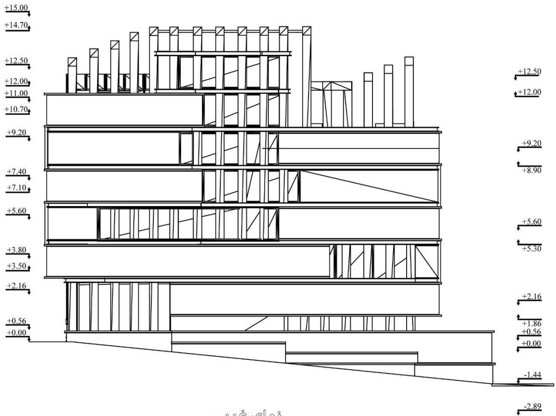
نمای غربی
