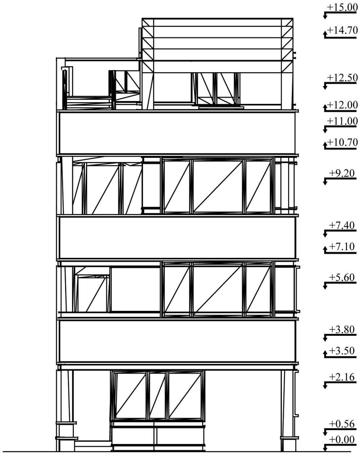
نما شمالی
