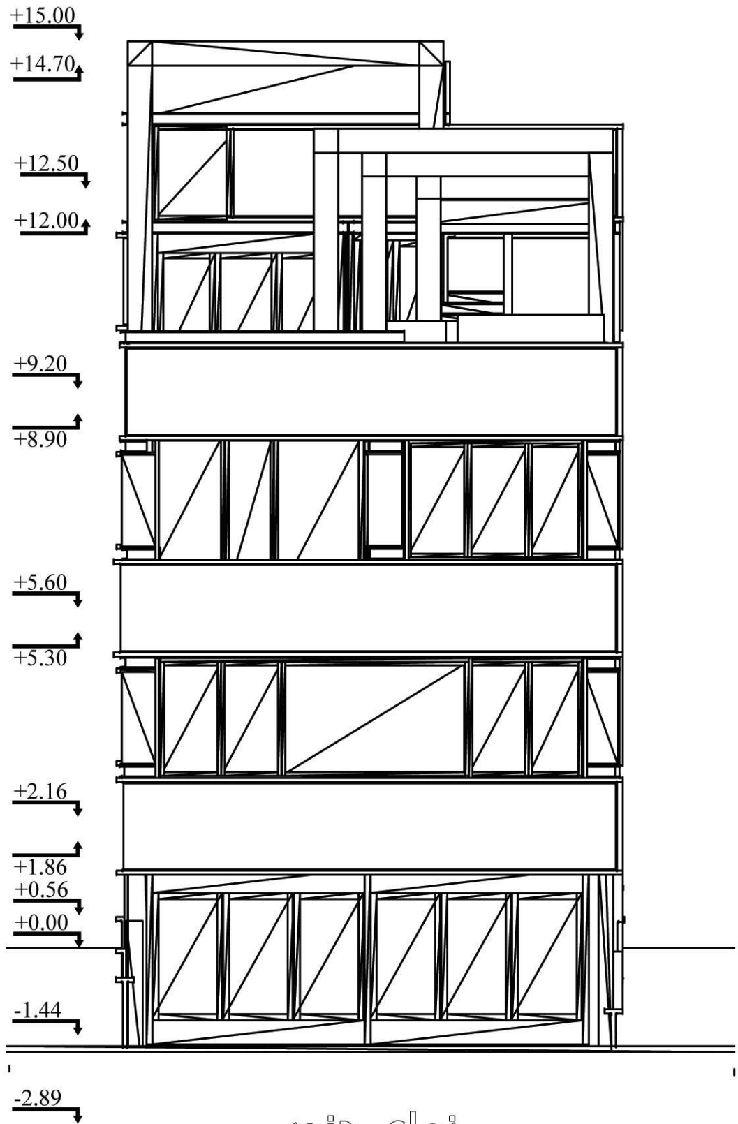
نمای جنوبی
