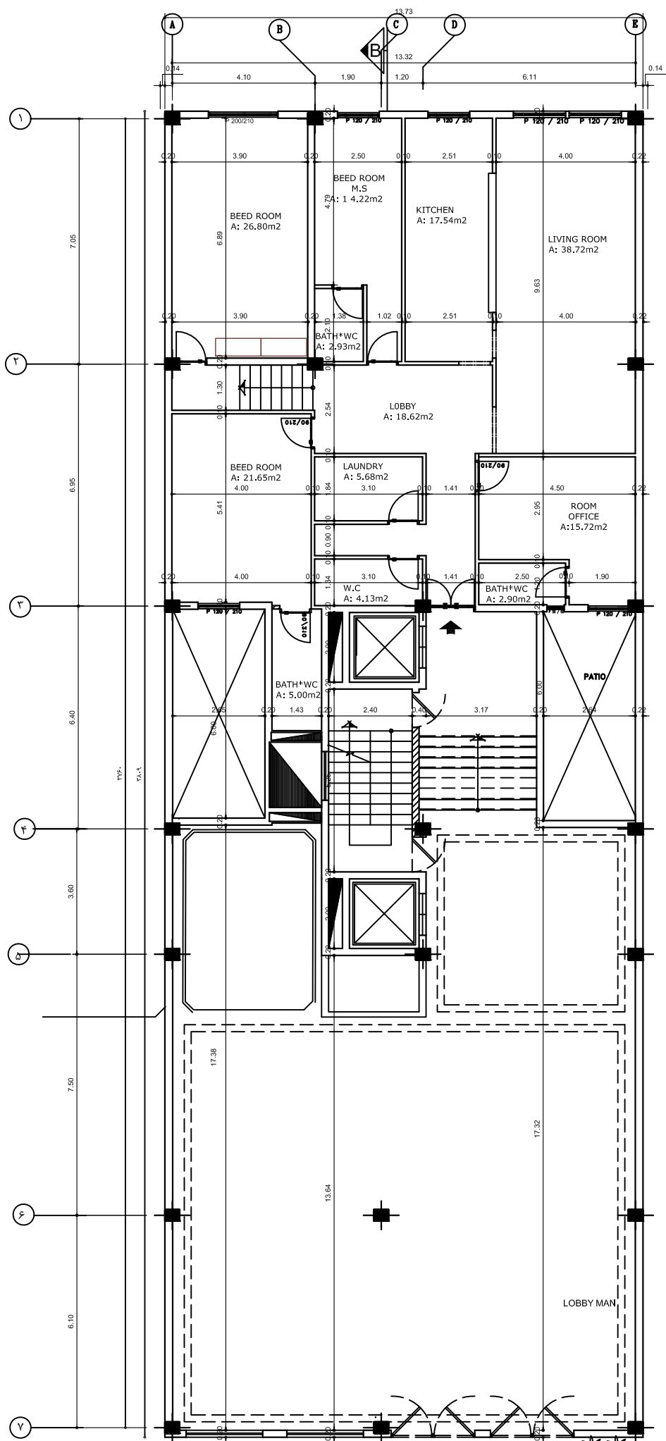
پلان اندازه گذاری طبقه همکف واحد شمالی
