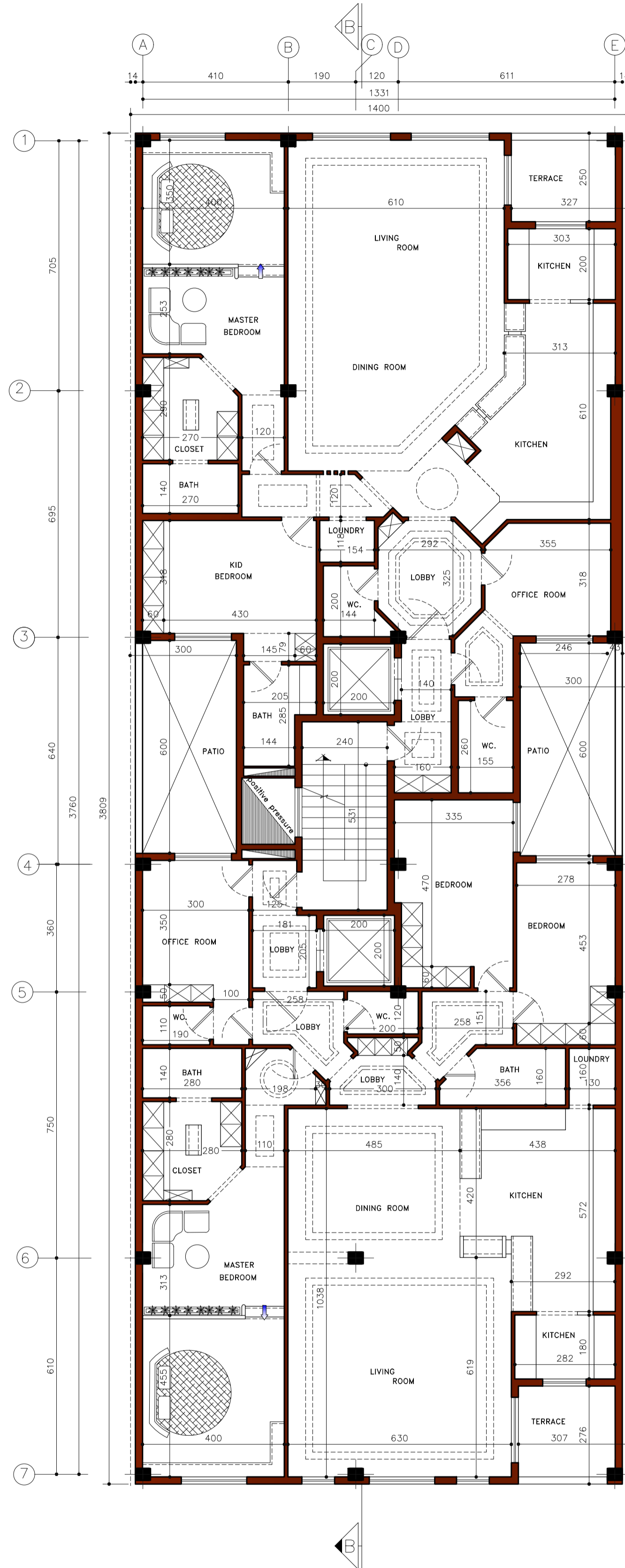
پلان اندازه گذاری طبقات SC. 1:100
