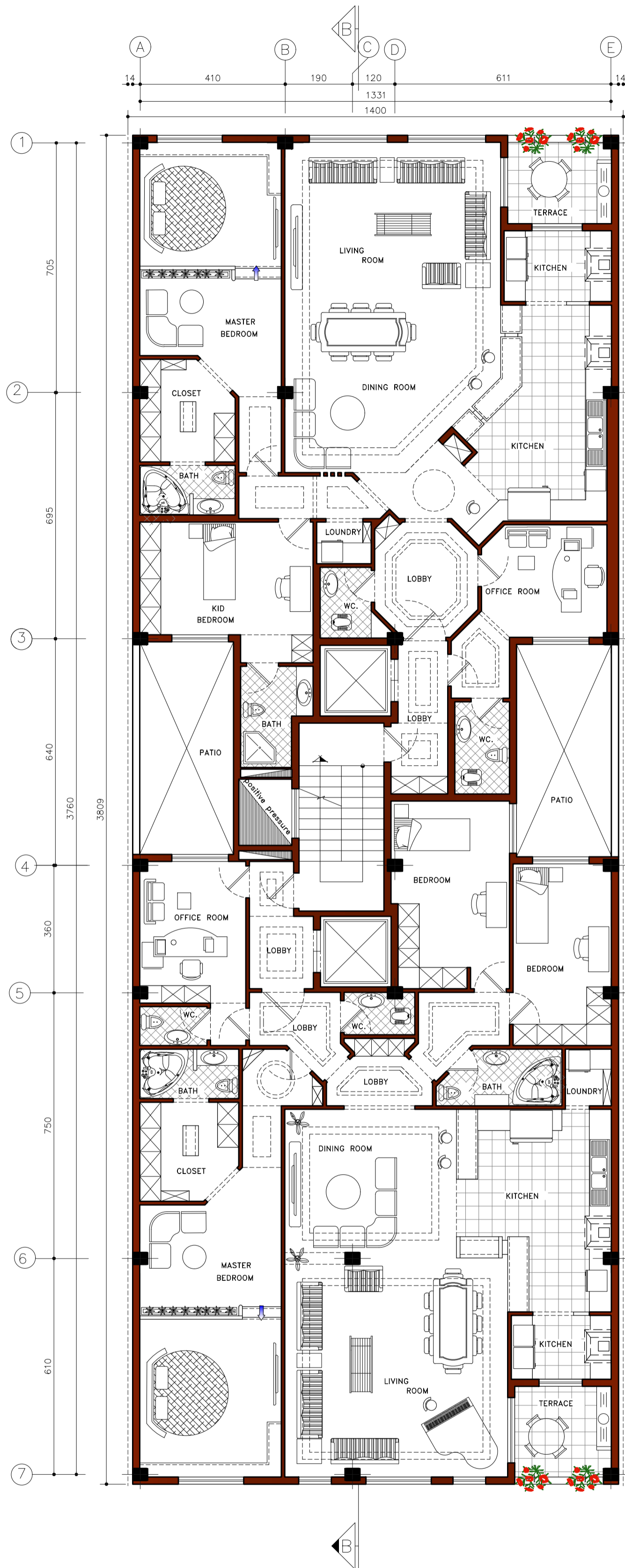
پلان مبلمان طبقات SC. 1:100
