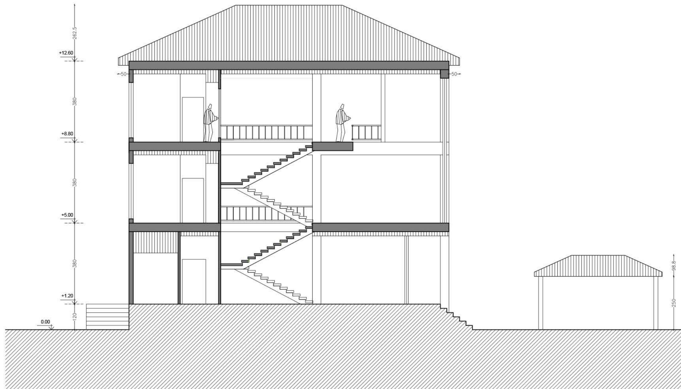
برش A-A
