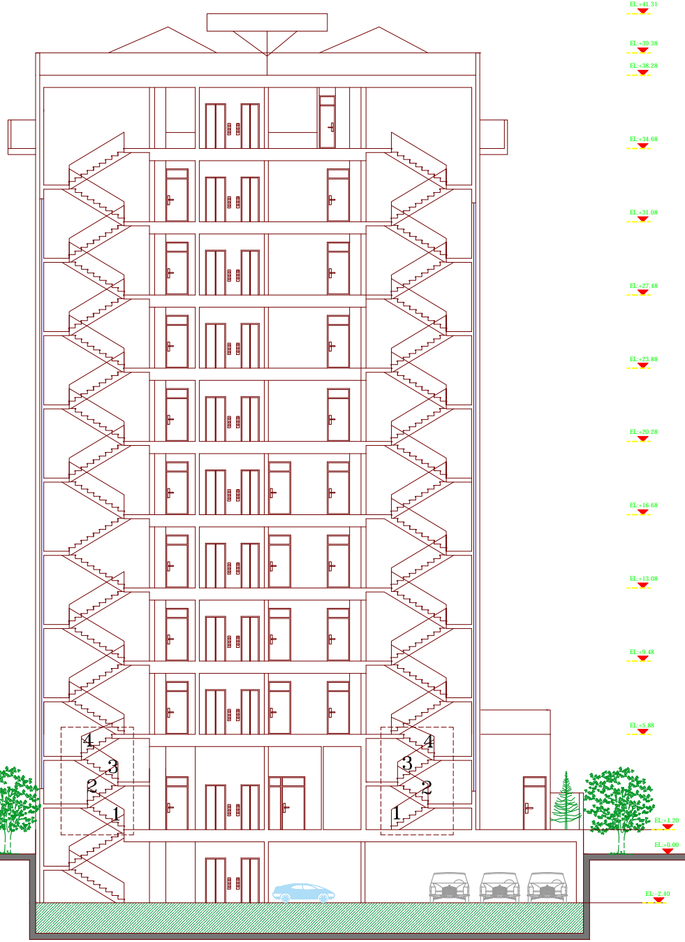
Section A-A
