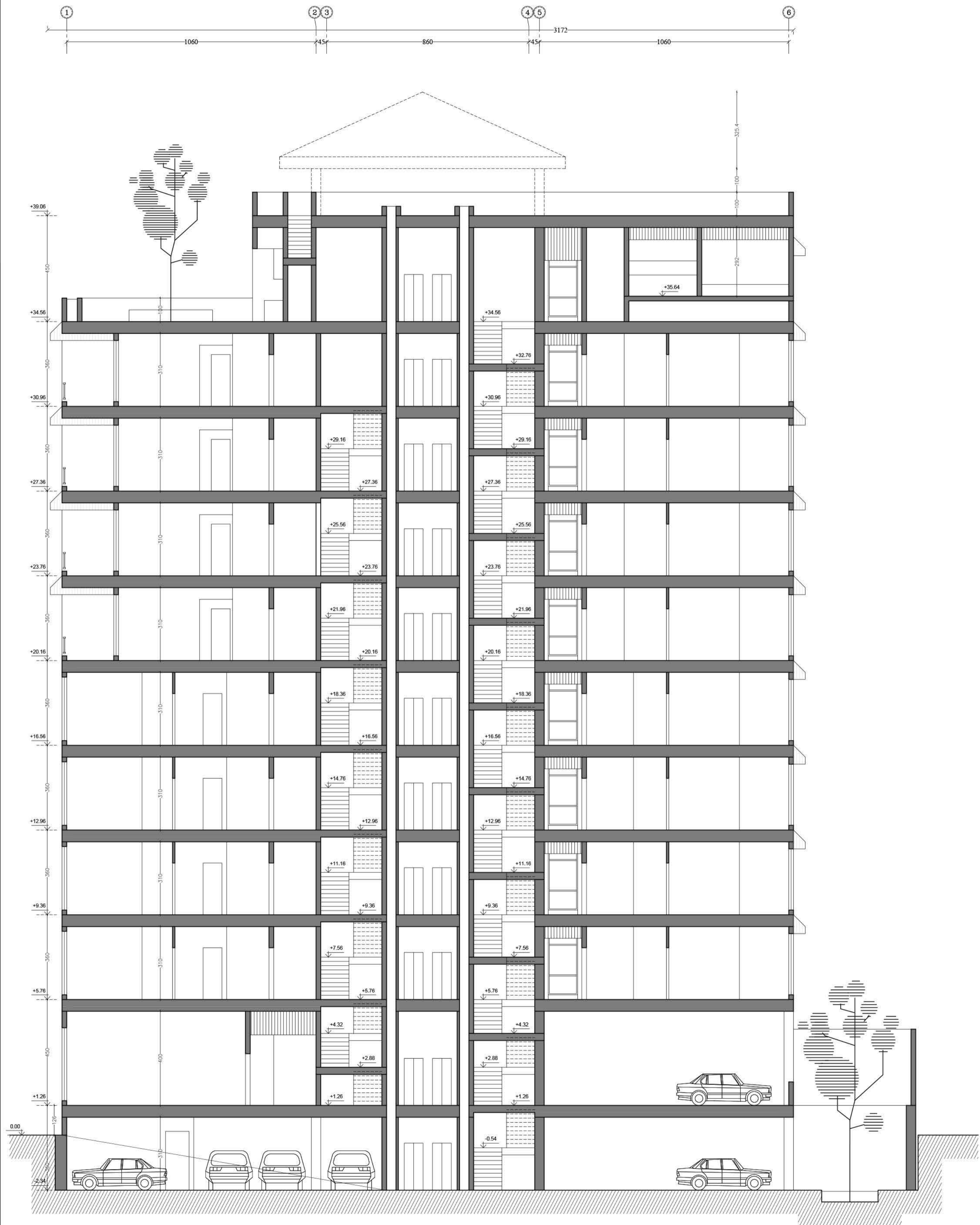
برش B-B
