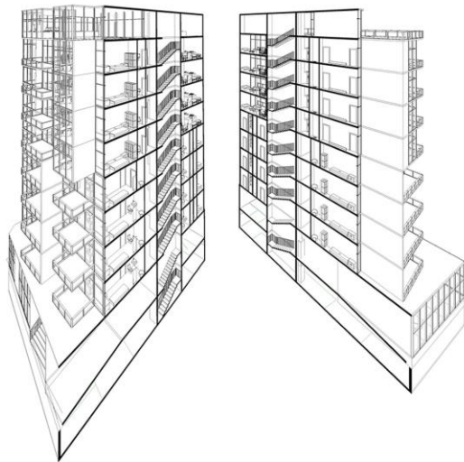
برش A
