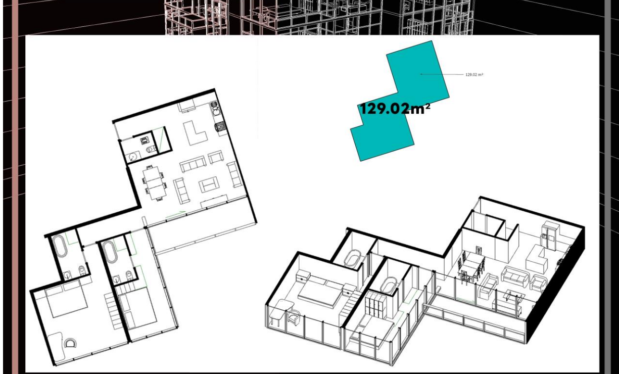
مساحت پلان های واحد های دو خوابه طبقه پنجم تا هشتم
