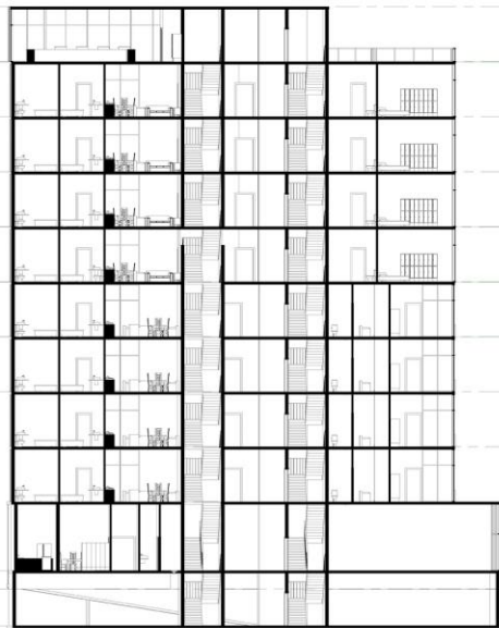
برش A
