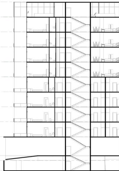
برش B
