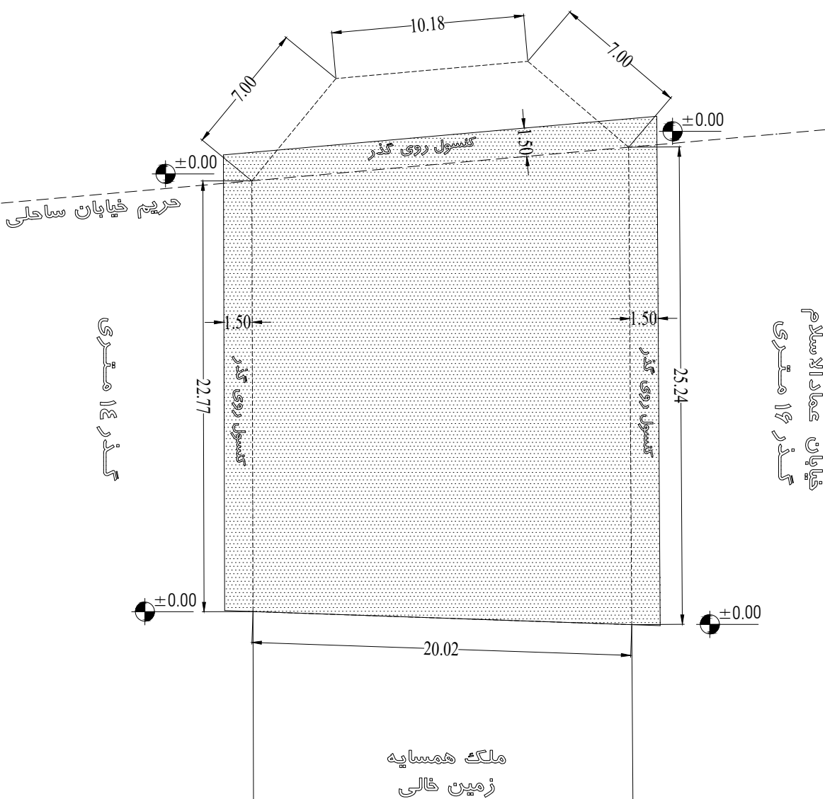
1 Site Plan 1:100
