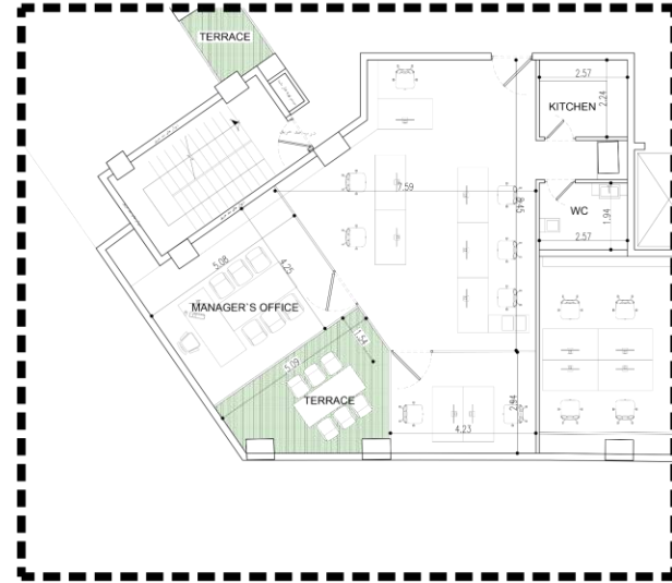
پلان تیپ دوم واحد اداری جنوب غربی
