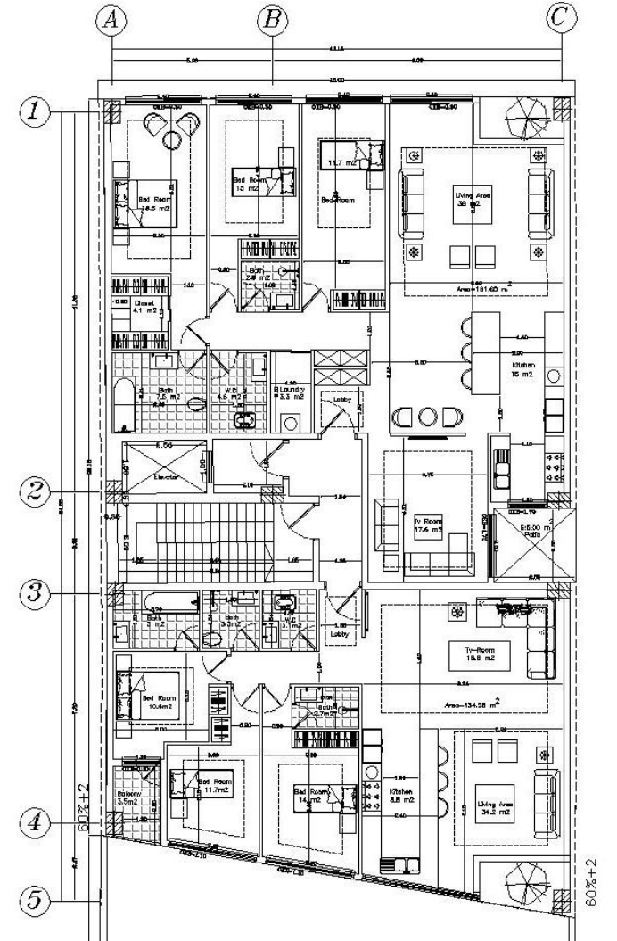
پلان طبقه سوم
