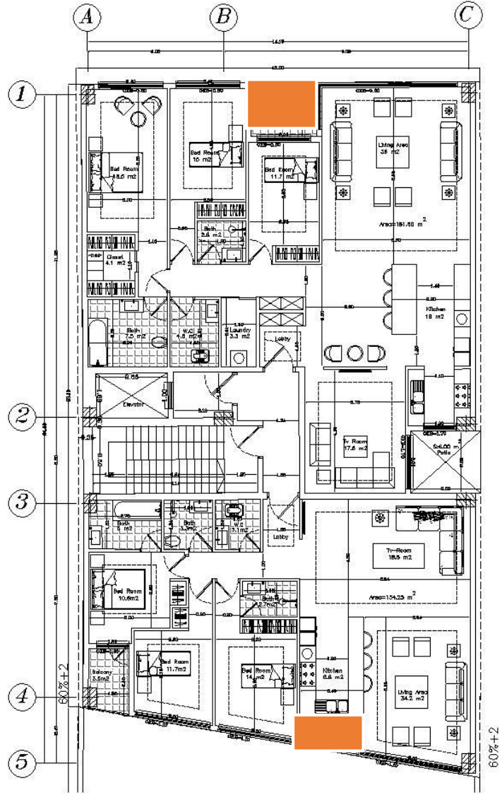
پلان طبقات اول - چهارم - پنجم
