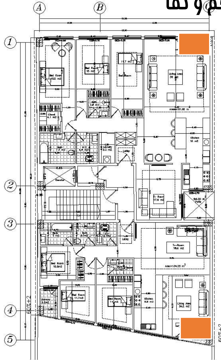
پلان طبقه دوم
