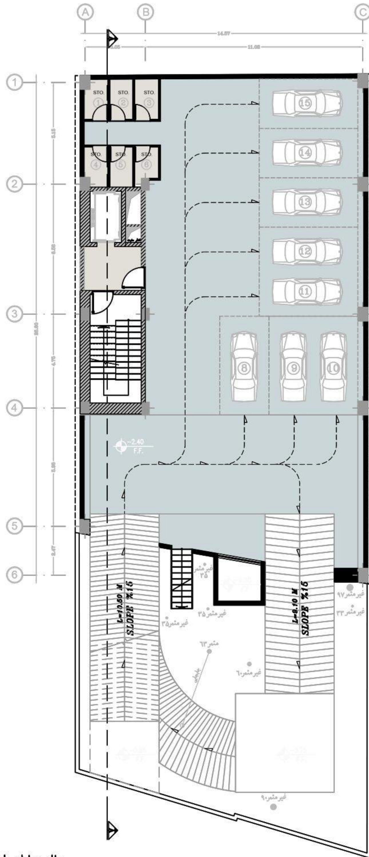
پلان مبلمان طبقه زیرزمین اول
