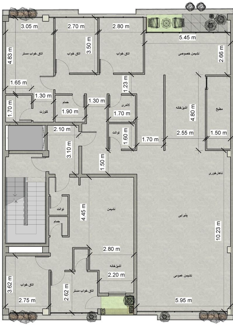
پلان مترائز طبقات
