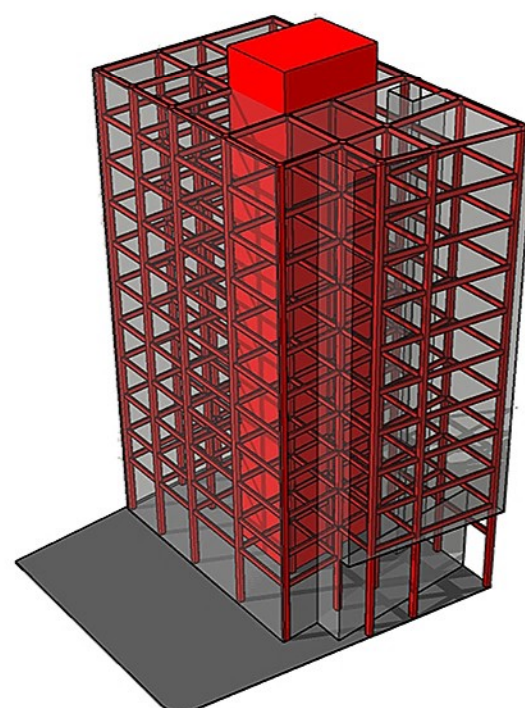
۳ طراحی عناصر سازه ای در حالت اپتیوموم
