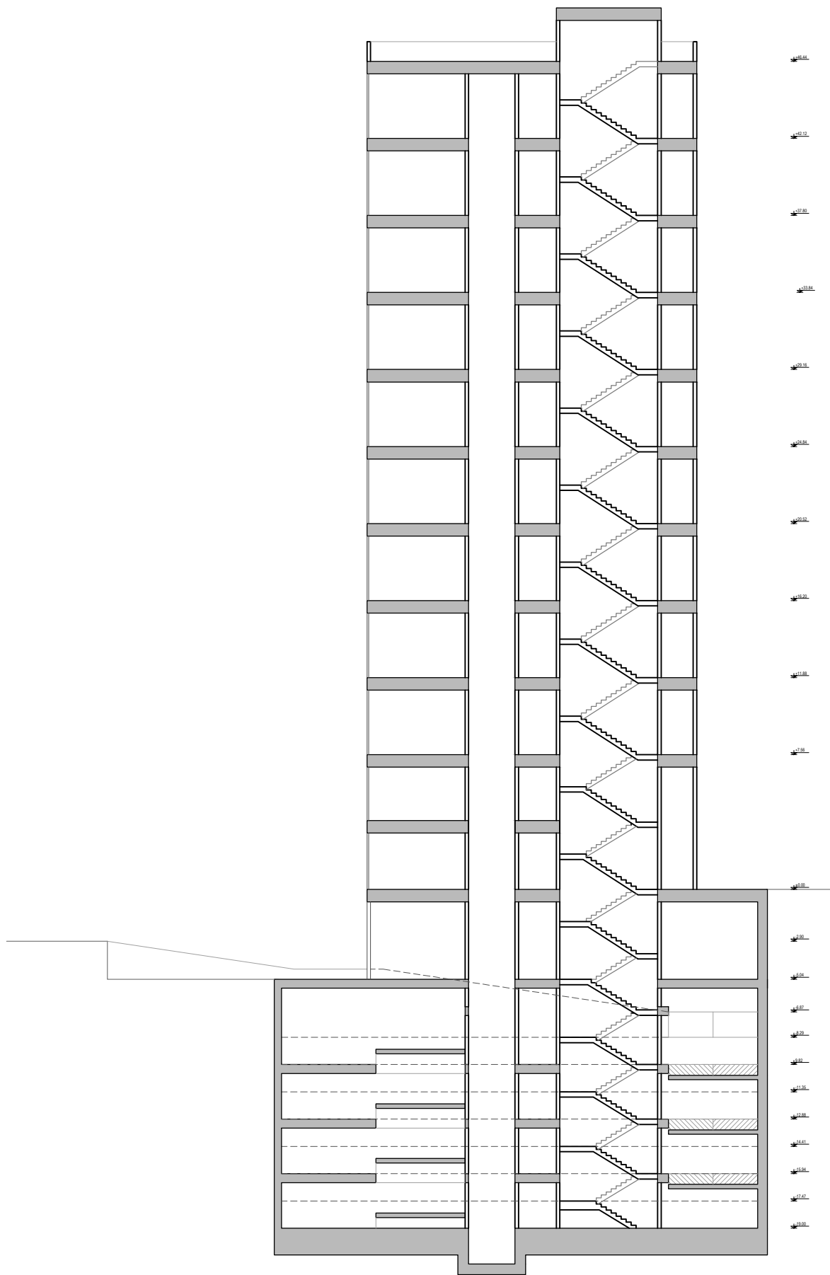
SECTION A-A
