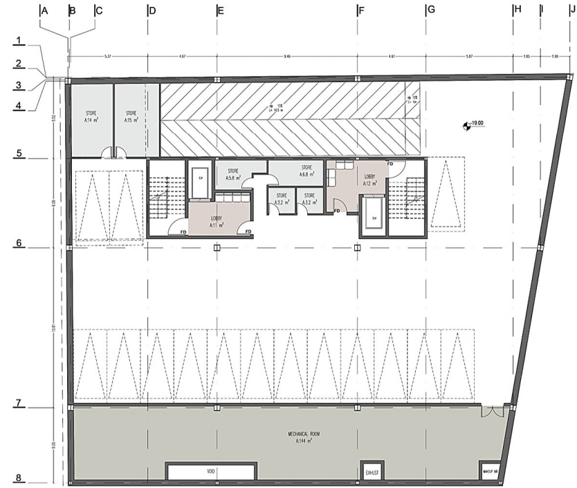
پلان زیر زمین ۰-
