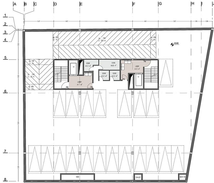
پلان زیر زمین ۳ و ۴-
