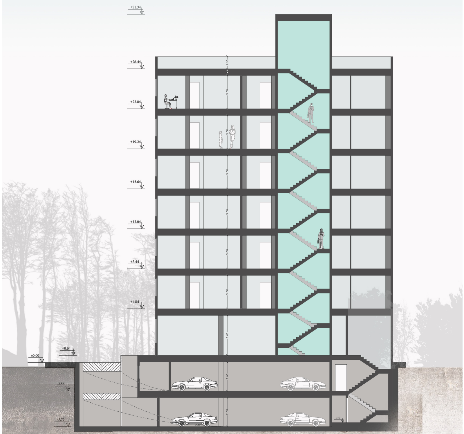
SEC A-A 1:100
