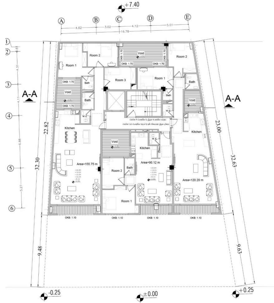
پلان تپ طبقات
