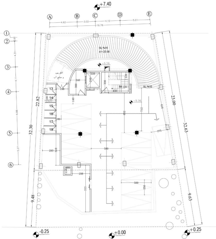
پلان طبقه پارکینگ ۲-
