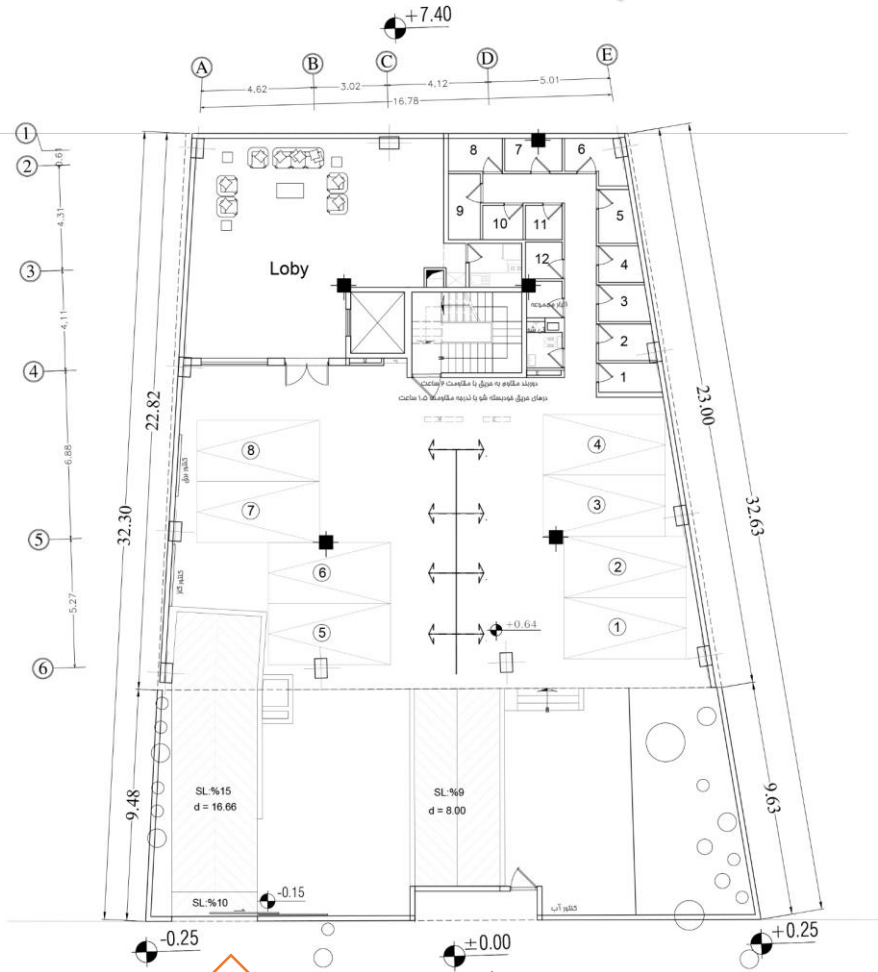
پلان طبقه همکف
