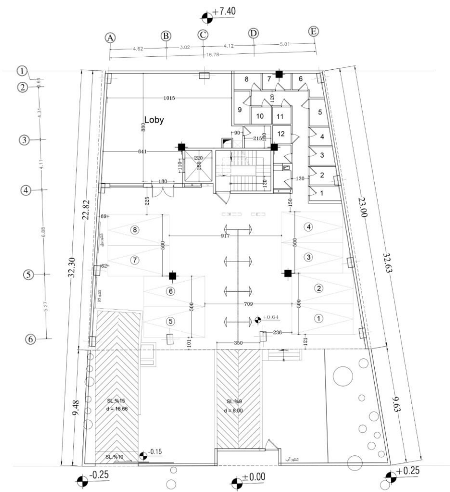
پلان طبقه همکف
