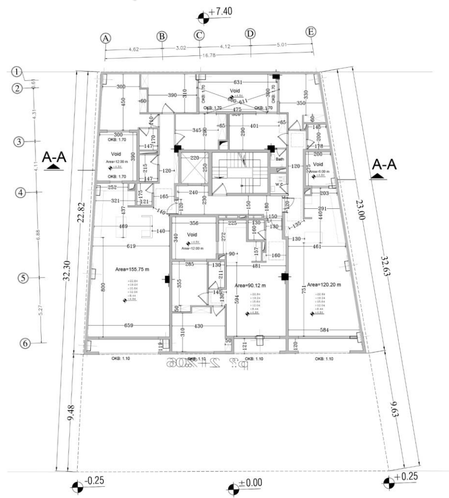
پلان تیب طبقات
