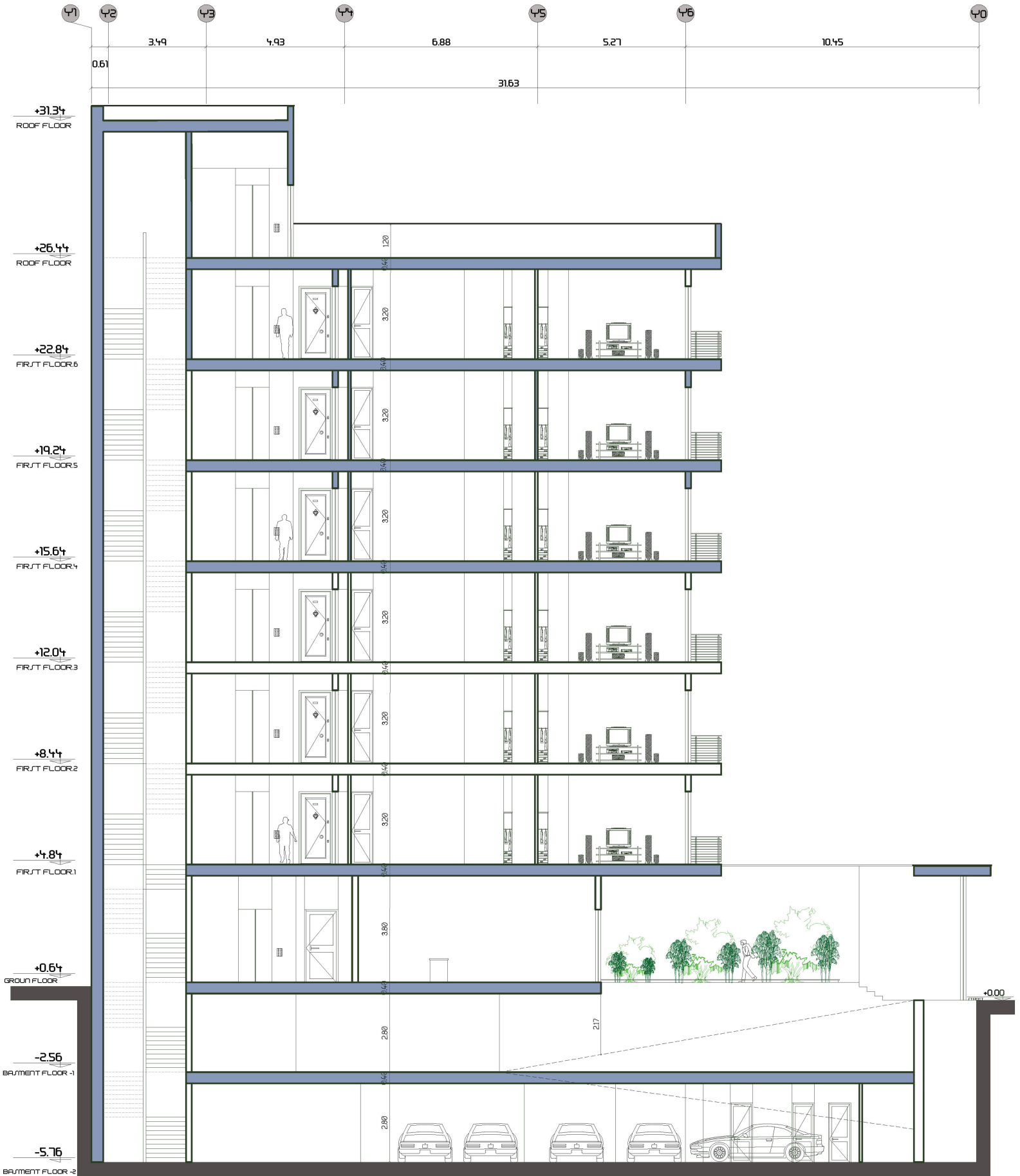
SEC A-A SC:1:100
