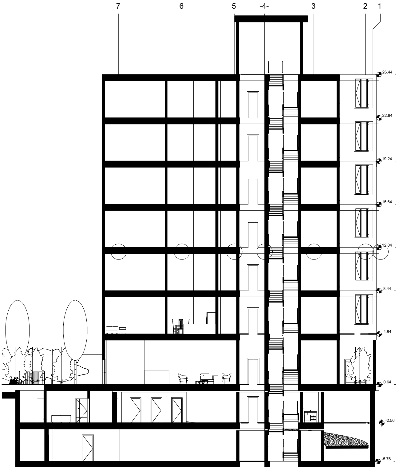
B-B مقطع
