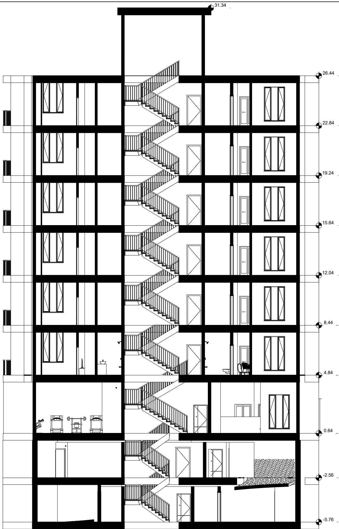
A-A مقطع
