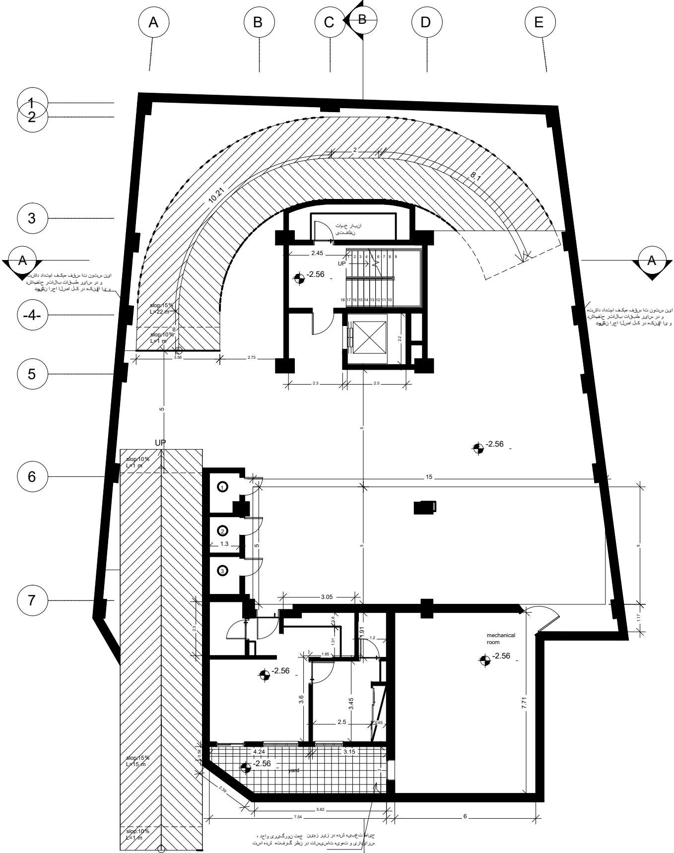
پلان اندازه گذاری زیرزمین اول
