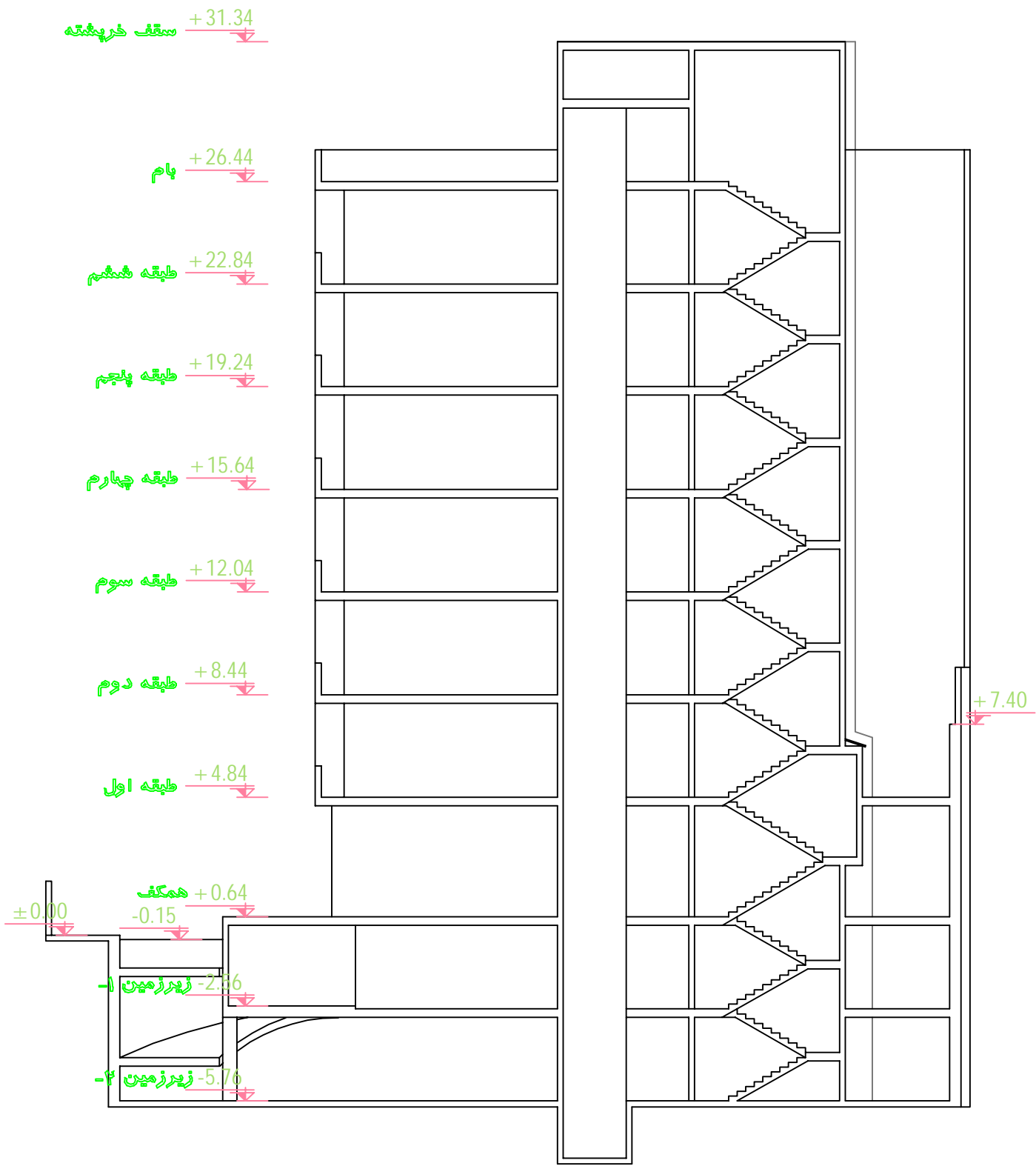
A-A Section
