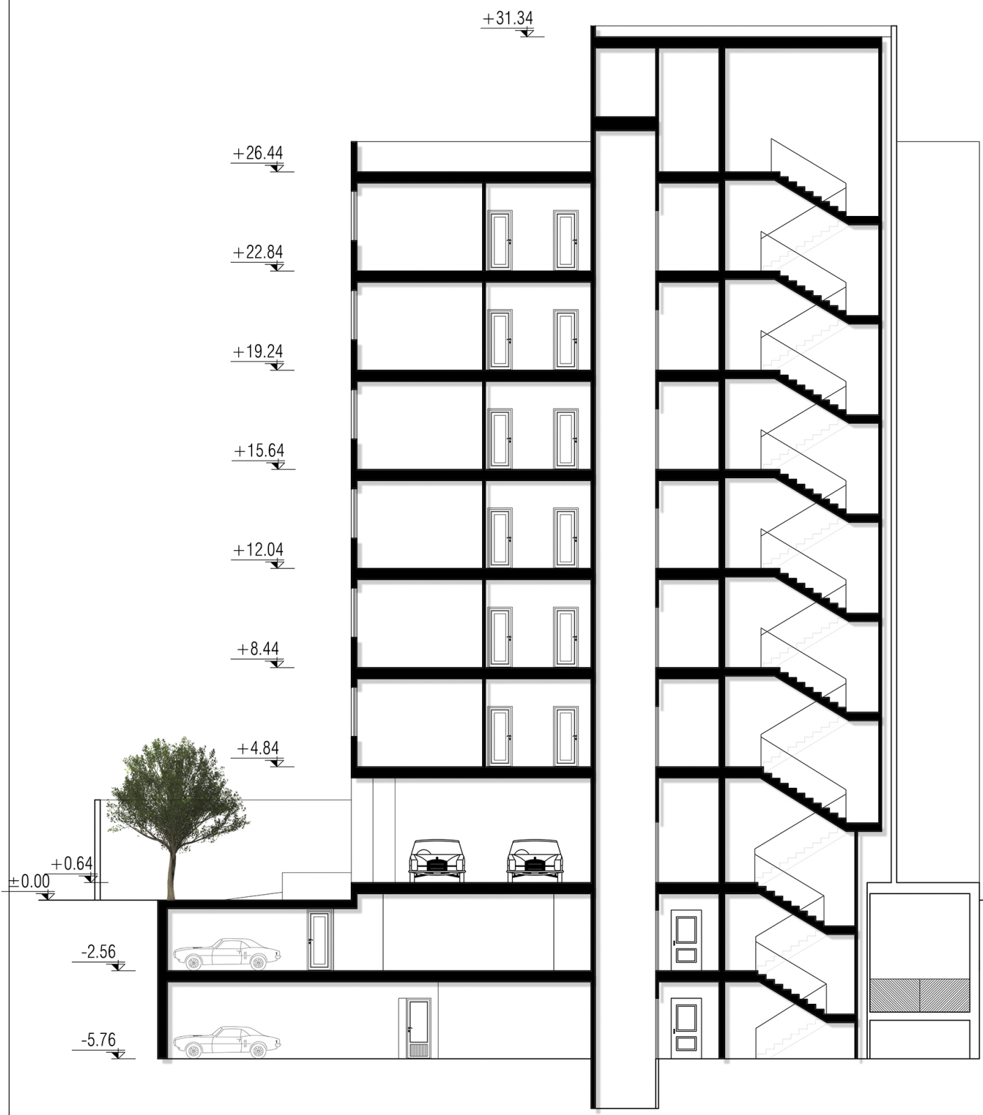
مقطع A-A SC:1/100
