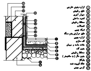
جزئیات عایق حرارتی کف
