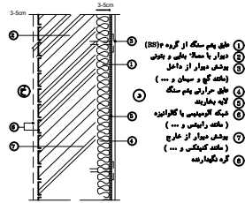
جزئیات عایق حرارتی دیوار خارجی
