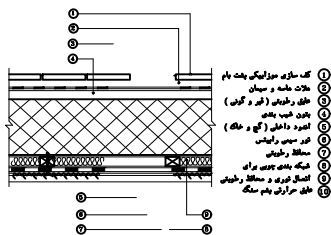
جزئیات عایق حرارتی بام
