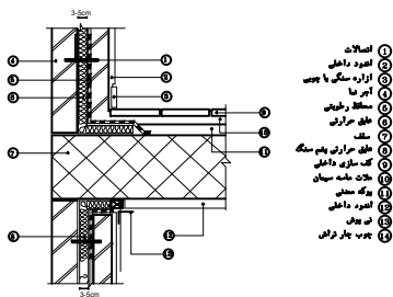
جزئیات عایق حرارتی دیوار جانبی
