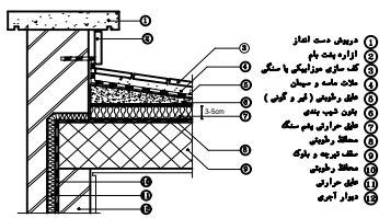
جزئیات عایق حرارتی گوشه بام به دیوار جانبی
