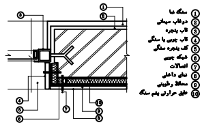
جزئیات عایق حرارتی دیوار به پنجره
